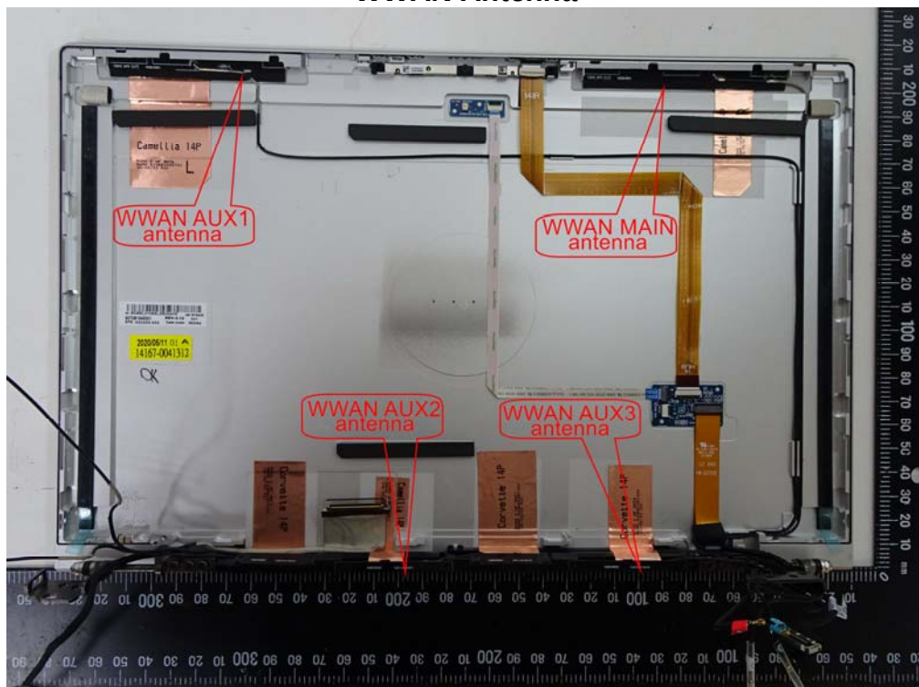
WWAN Antenna
