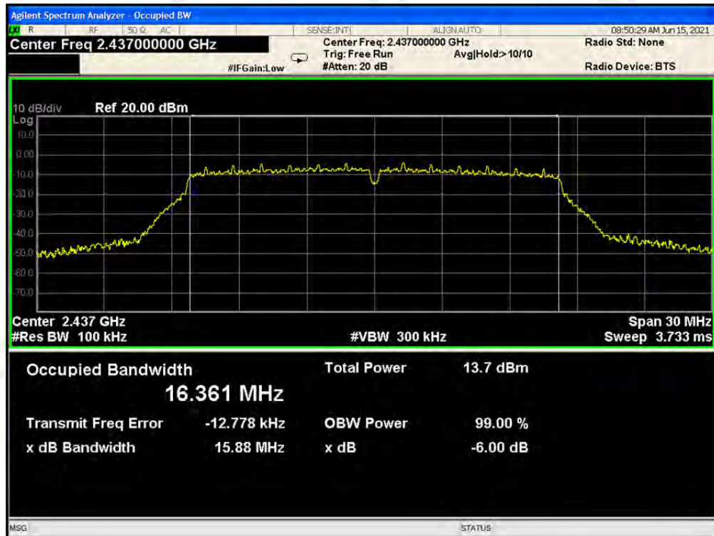
CH6: 2437MHz
