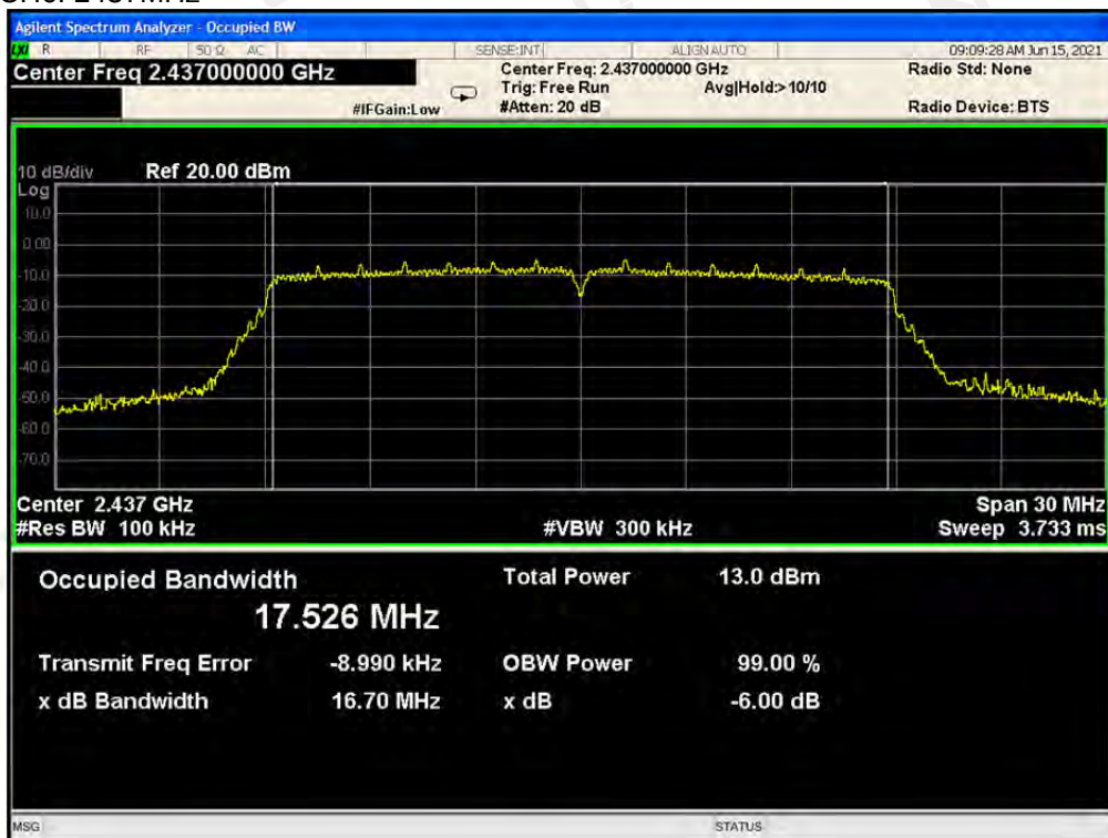
CH6: 2437MHz
