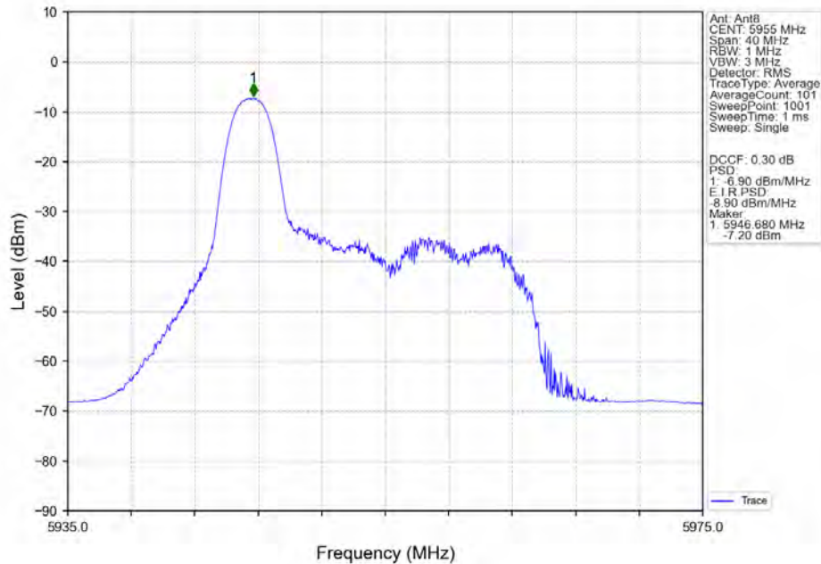
802.11ax(HEW20) LCH_5955MHz RU26 Left MIMO NTVN
