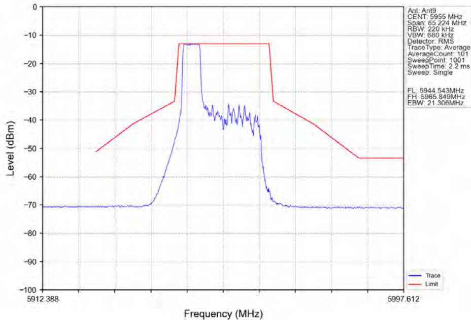
802.11ax(HEW20) LCH 5955MHz RU106 Left Ant9 NTN
