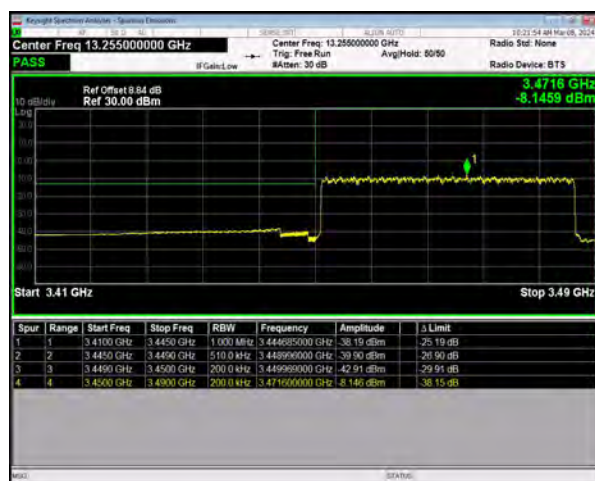
n77(3450-3550) SCS=30kHz DFT_QPSK BW=40MHz
