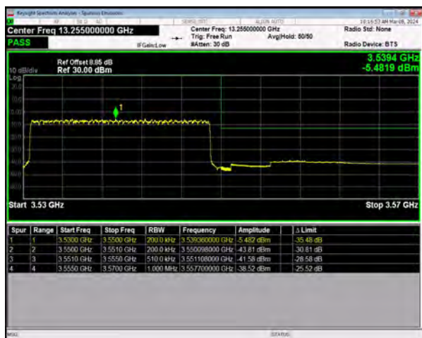
n77(3450-3550) SCS=30kHz DFT_BPSK BW=20MHz
