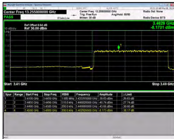
n77(3450-3550) SCS=30kHz DFT_BPSK BW=40MHz
