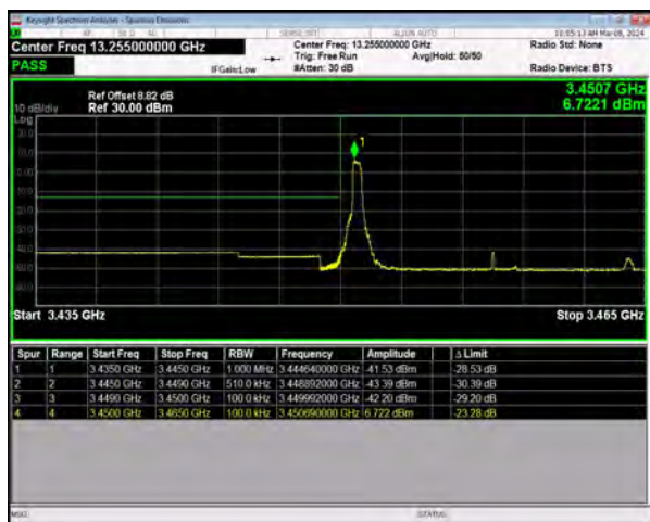
n77(3450-3550) SCS=30kHz DFT_16QAM BW=15MHz
