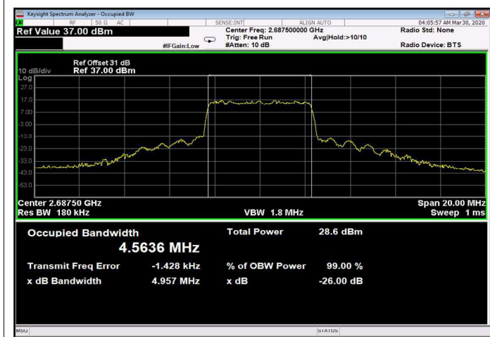
Figure 349: 64QAM 5MHz B.W.; 2687.5MHz, 15kHz Output
