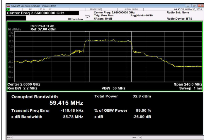
Figure 391: 64QAM 60MHz B.W.; 2660.0MHz, 30kHz Output
