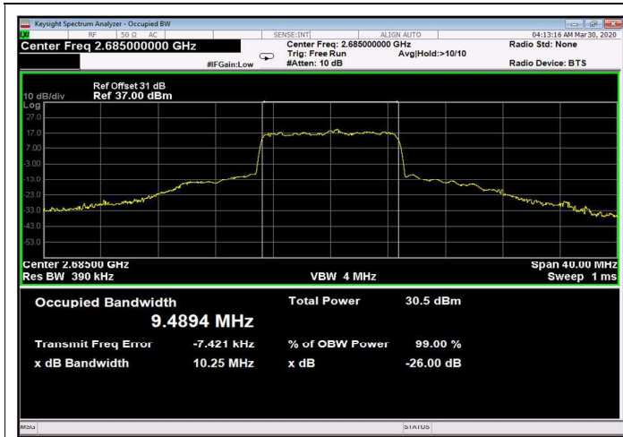
Figure 357: 64QAM 10MHz B.W.; 2685.0MHz, 15kHz Output
