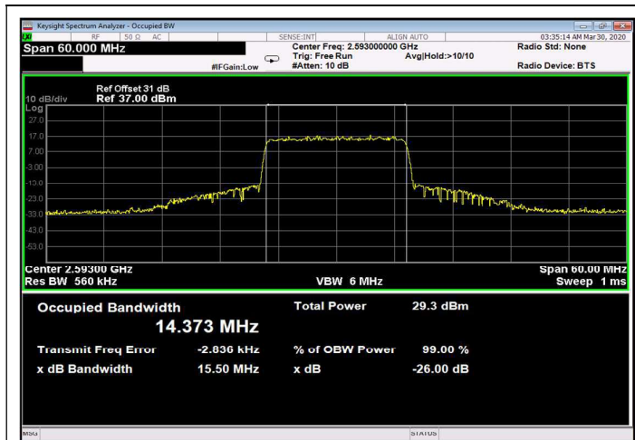
Figure 363: 64QAM 15MHz B.W.; 2593.0MHz, 15kHz Output
