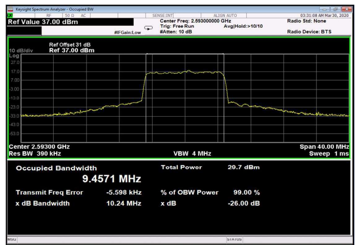
Figure 354: 64QAM 10MHz B.W.; 2593.0MHz, 15kHz Output
