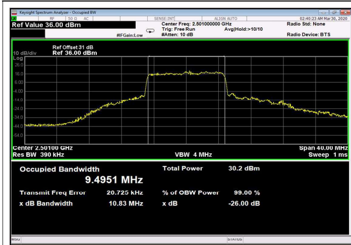
Figure 351: 64QAM 10MHz B.W.; 2501.0MHz, 15kHz Output
