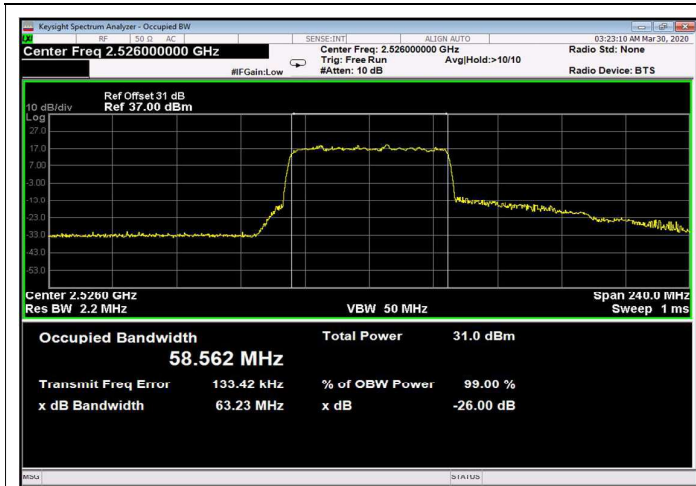
Figure 387: 64QAM 60MHz B.W.; 2526.0MHz, 30kHz Output
