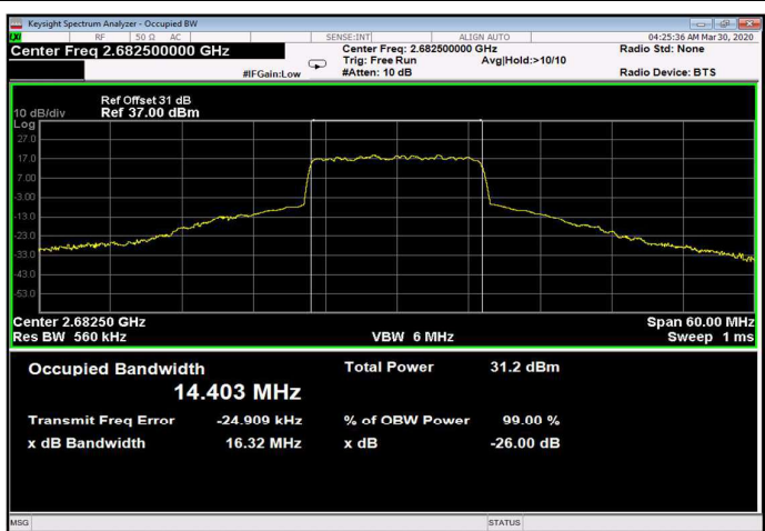
Figure 366: 64QAM 15MHz B.W.; 2682.5MHz, 15kHz Output
