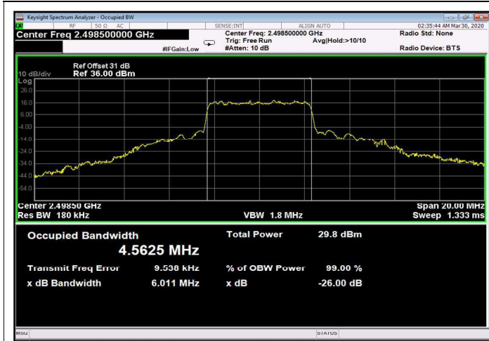
Figure 345: 64QAM 5MHz B.W.; 2498.5MHz, 15kHz Output
