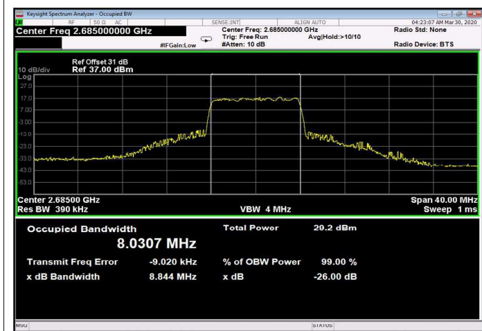
Figure 359: 64QAM 10MHz B.W.; 2685.0MHz, 60kHz Output
