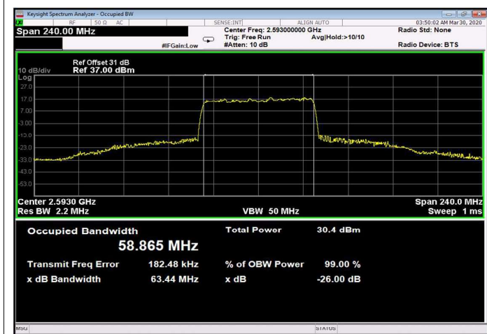
Figure 389: 64QAM 60MHz B.W.; 2593.0MHz, 30kHz Output
