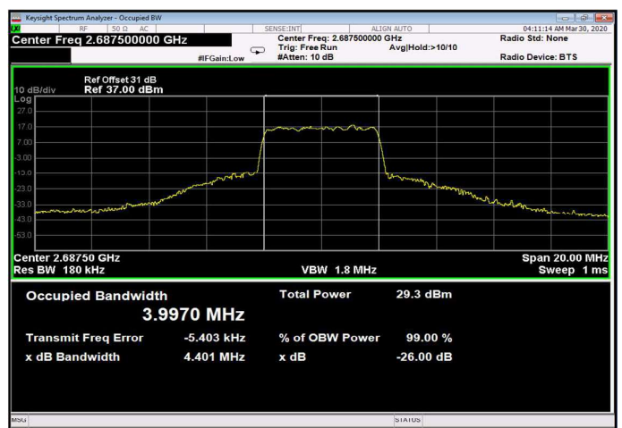
Figure 350: 64QAM 5MHz B.W.; 2687.5MHz, 30kHz Output
