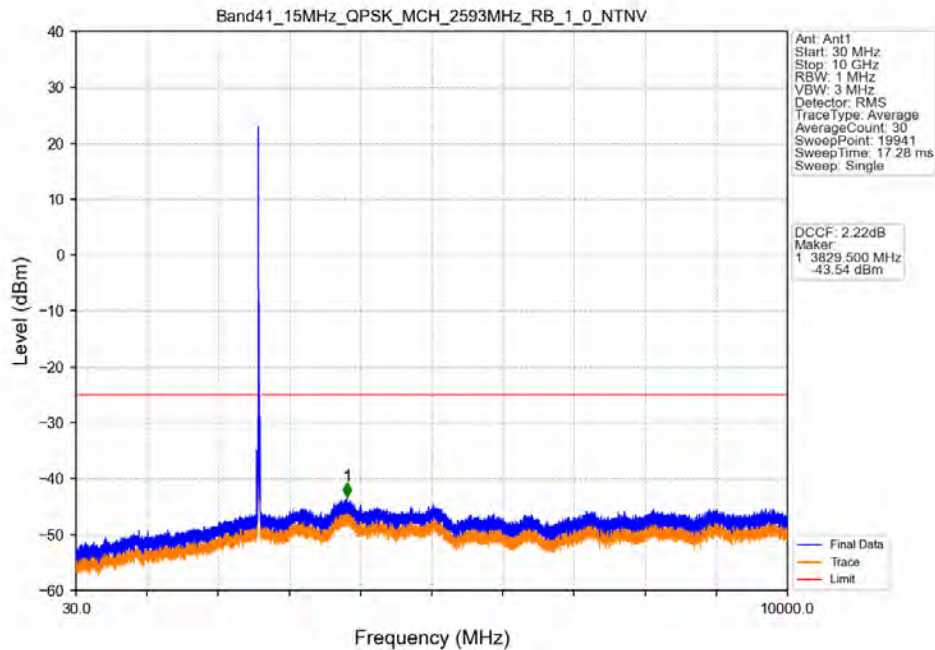
Band41_15MHz_QPSK_MCH_2593MHz_RB_1_0_NTNV
