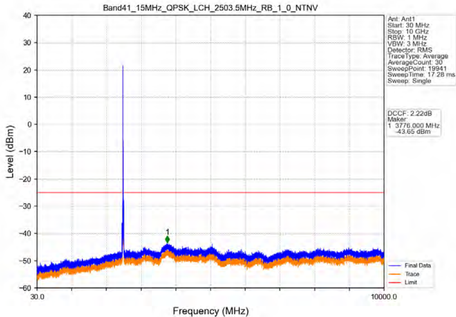
Band41_15MHz_QPSK_LCH_2503.5MHz_RB_1_0_NTNV
