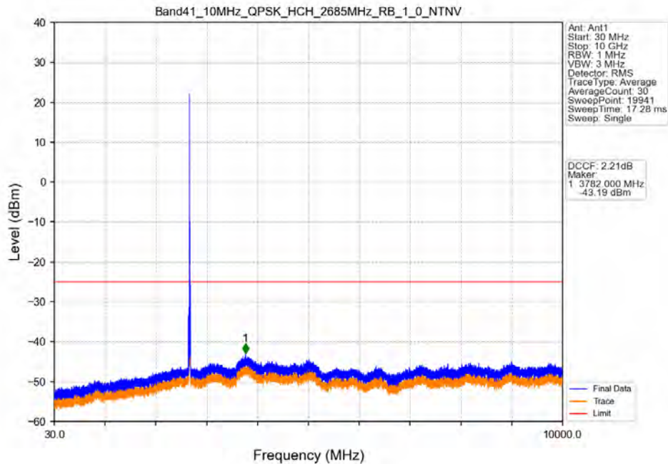
Band41_10MHz_QPSK_HCH_2685MHz_RB_1_0_NTNV
