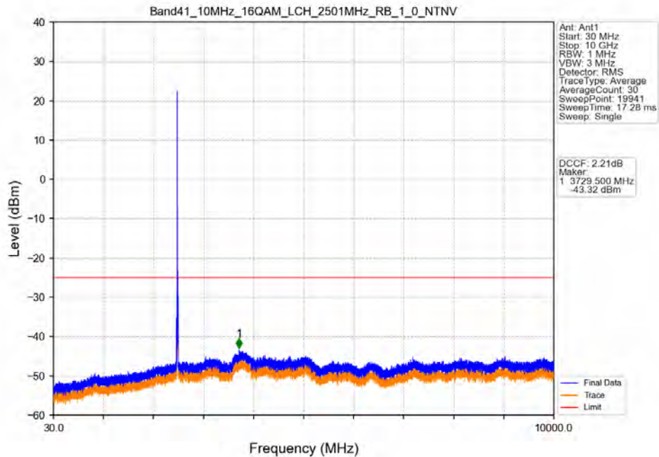
Band41_10MHz_16QAM_LCH_2501MHz_RB_1_0_NTNV
