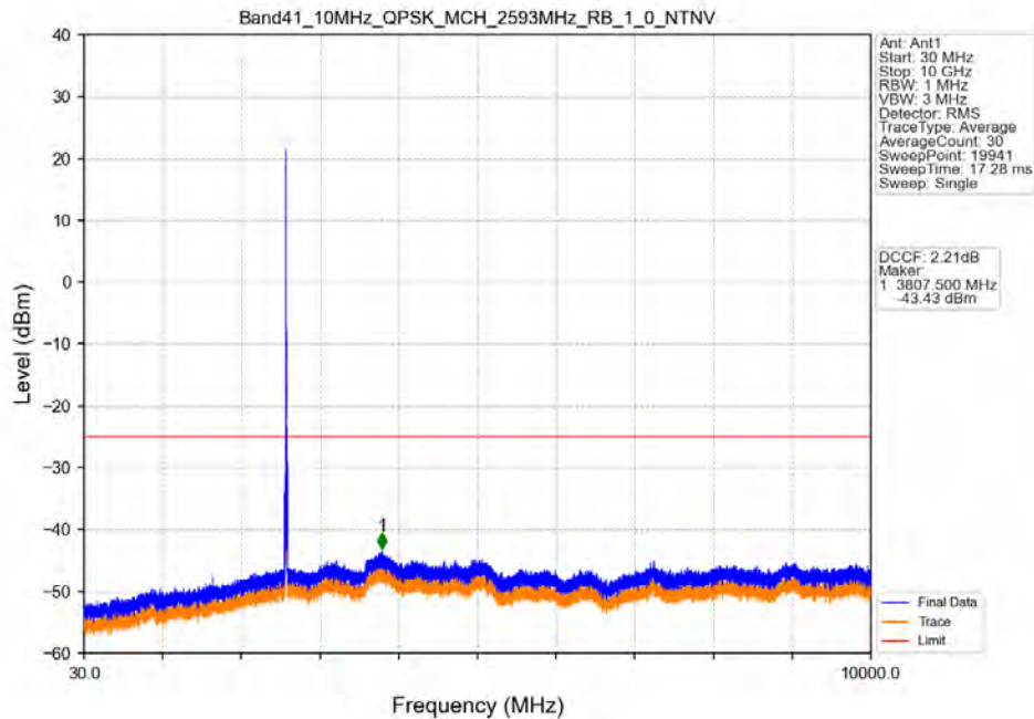
Band41_10MHz_QPSK_MCH_2593MHz_RB_1_0_NTNV
