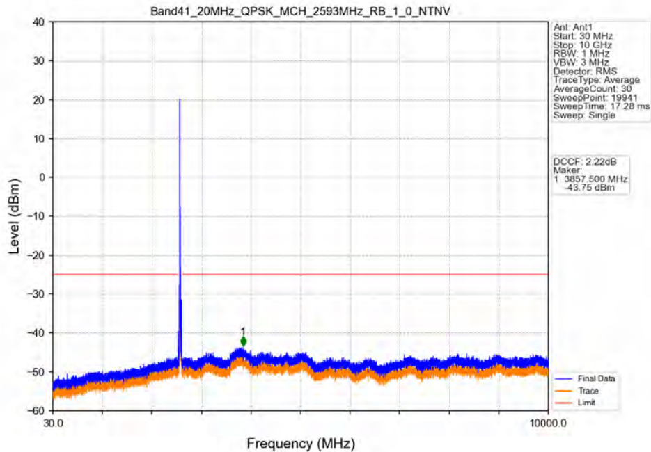
Band41_20MHz_QPSK_MCH_2593MHz_RB_1_0_NTNV
