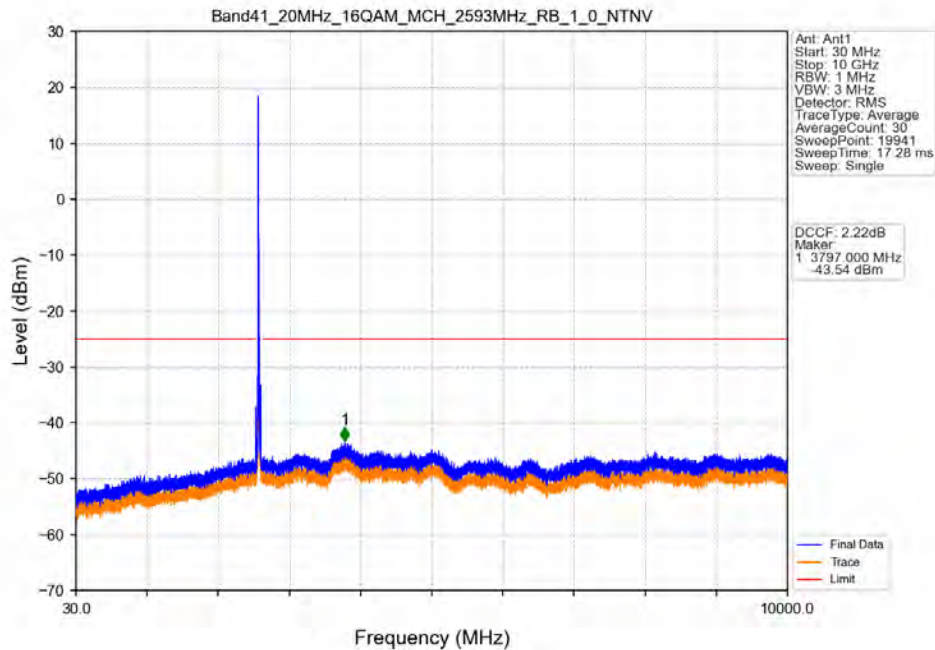
Band41_20MHz_16QAM_MCH_2593MHz_RB_1_0_NTNV
