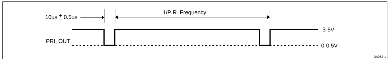
Figure 11. PRI_OUT / PRI_DPOS
