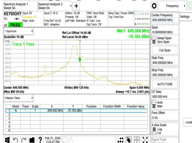
Band Edge_Band5_3MHz_QPSK_RB1_14_CH20635
