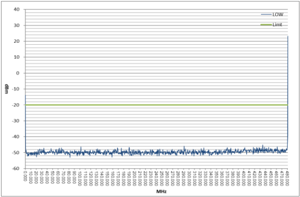
11K0F3E 9 KHz to Fc
