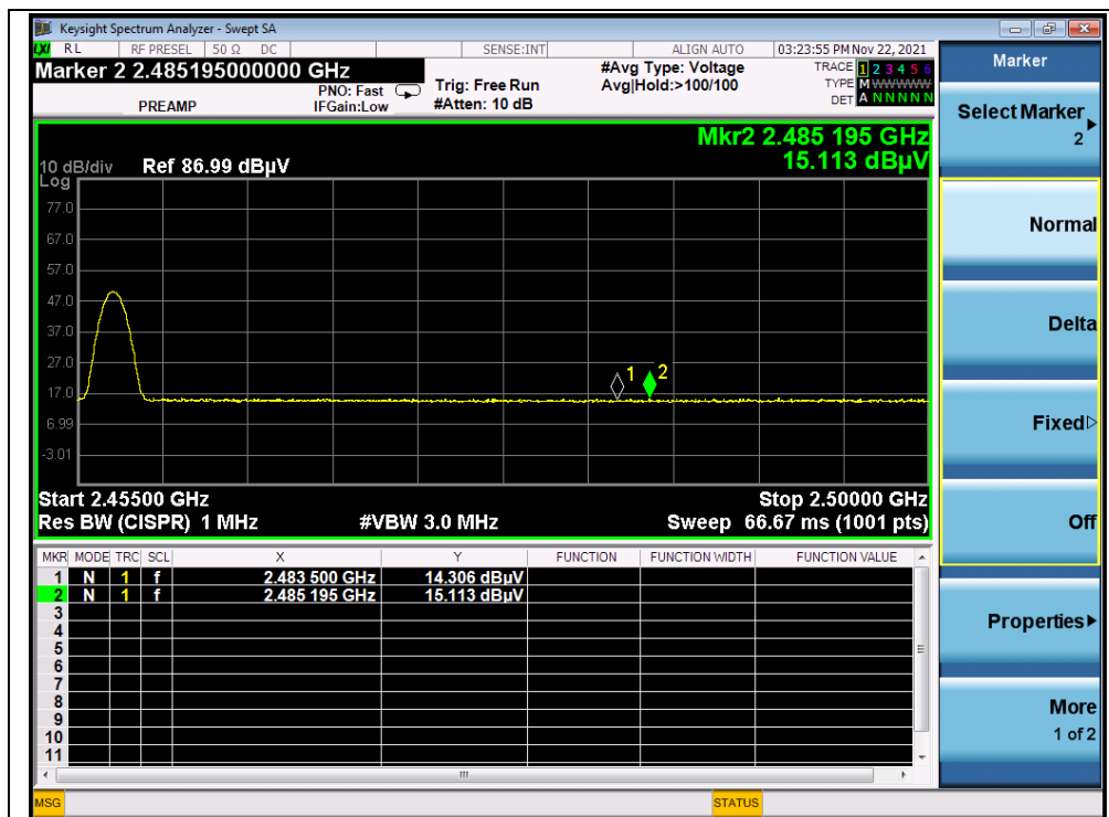
(AVERAGE, 2457MHz)
