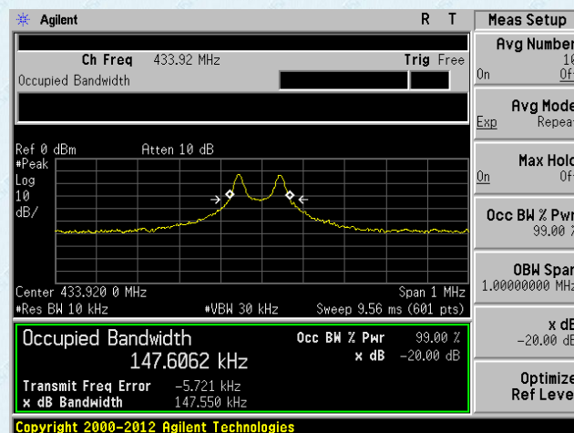
FSK
