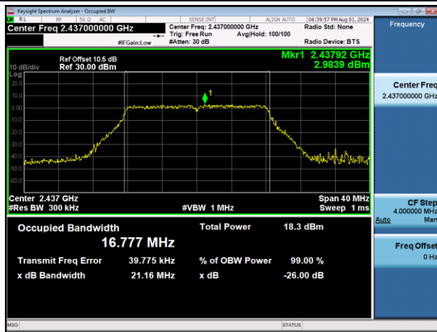
11G-Ant1-2437
