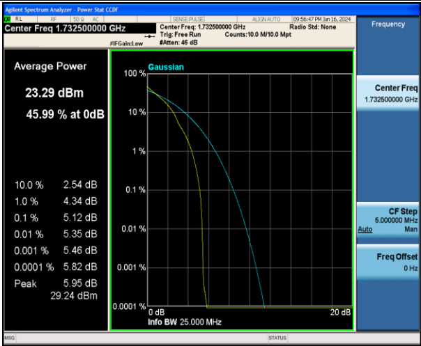
Band4-20MHz-QPSK-20175-1RB#0-PASS
