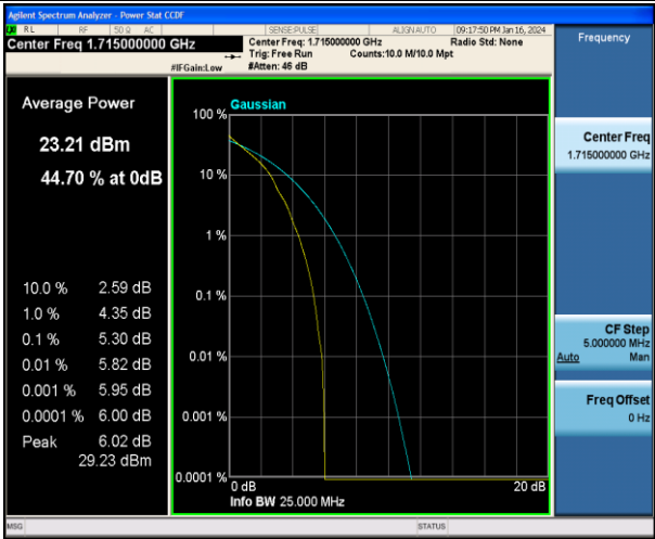
Band4-10MHz-QPSK-20000-1RB#0-PASS
