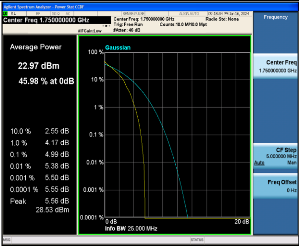
Band4-10MHz-QPSK-20350-1RB#0-PASS
