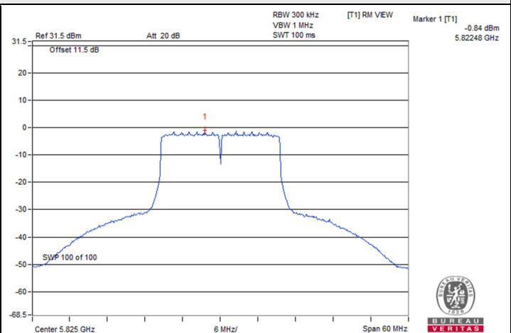
802.11be (EHT20) / Chain 3 : CH 165
