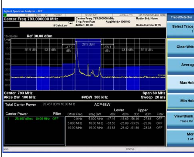
LTE Band 14 QPSK 1RB 10MHz CH Middle
