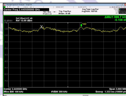
\pi /4DQPSK
