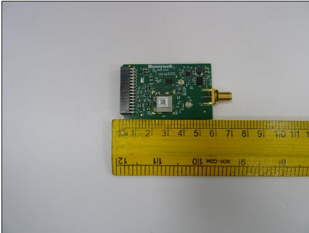
PM RF SOM PCB dimensional view
