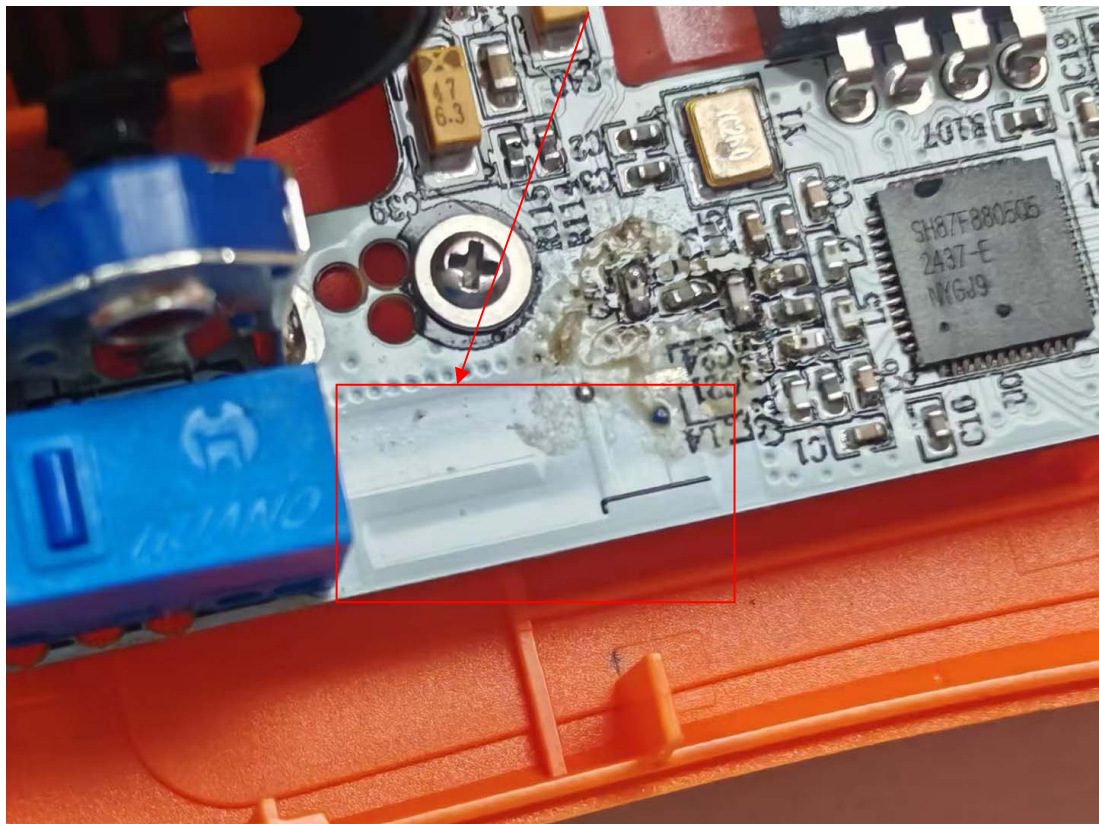
BLE&SRD Antenna
