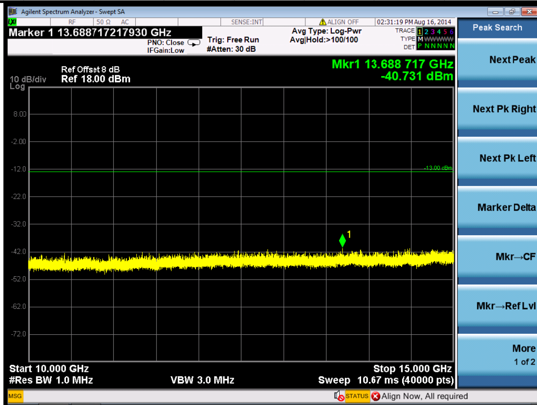
(Plot 5.5.1 D7: Idle WCDMA Band II)
