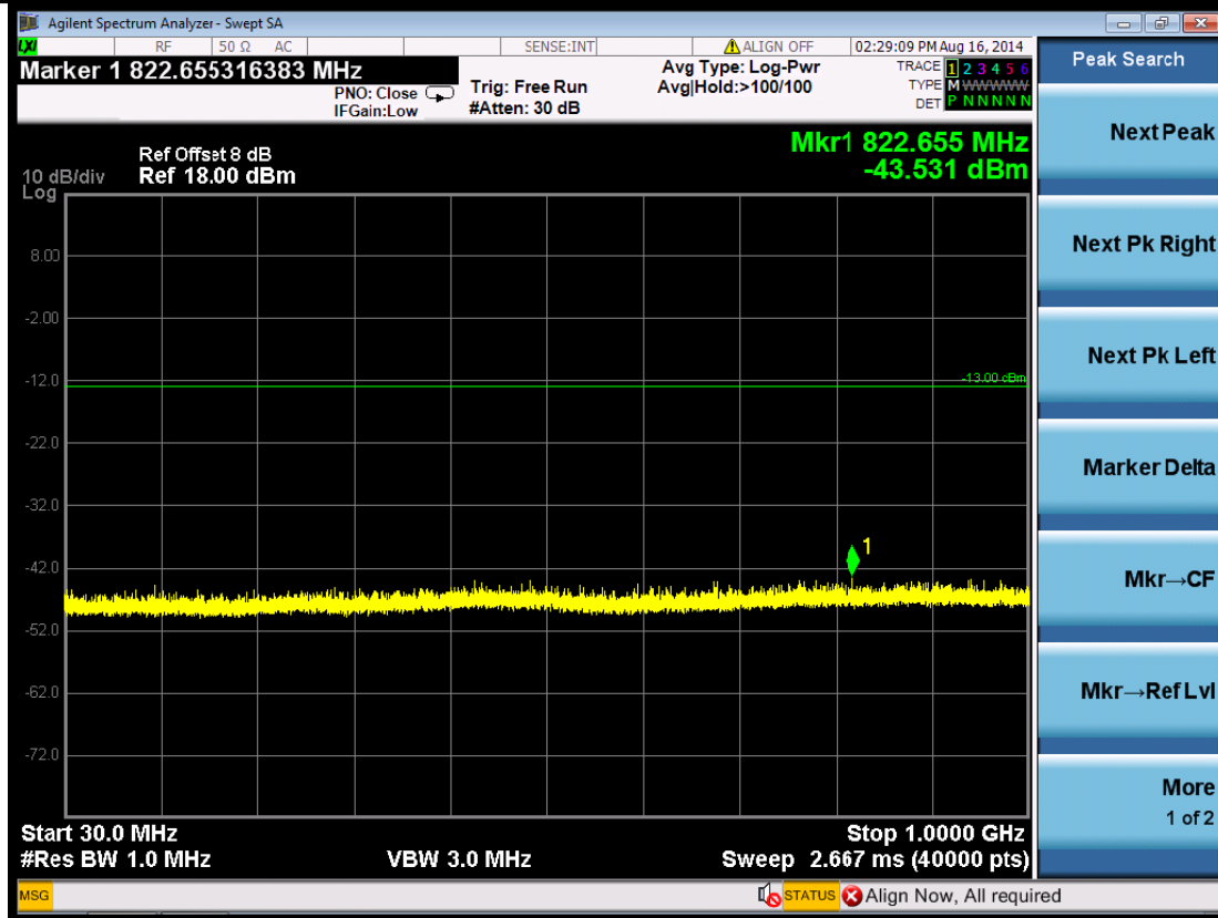
(Plot 4.5.1 D3: Idle WCDMA Band II)
