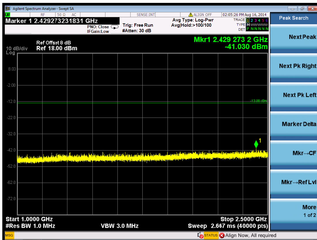
(Plot 5.5.3 D4: Idle WCDMA Band IV)
