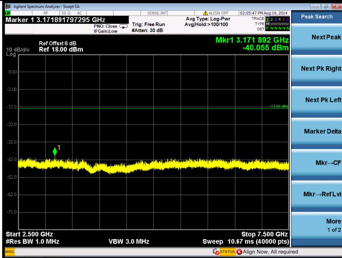
(Plot 5.5.3 D5: Idle WCDMA Band IV)
