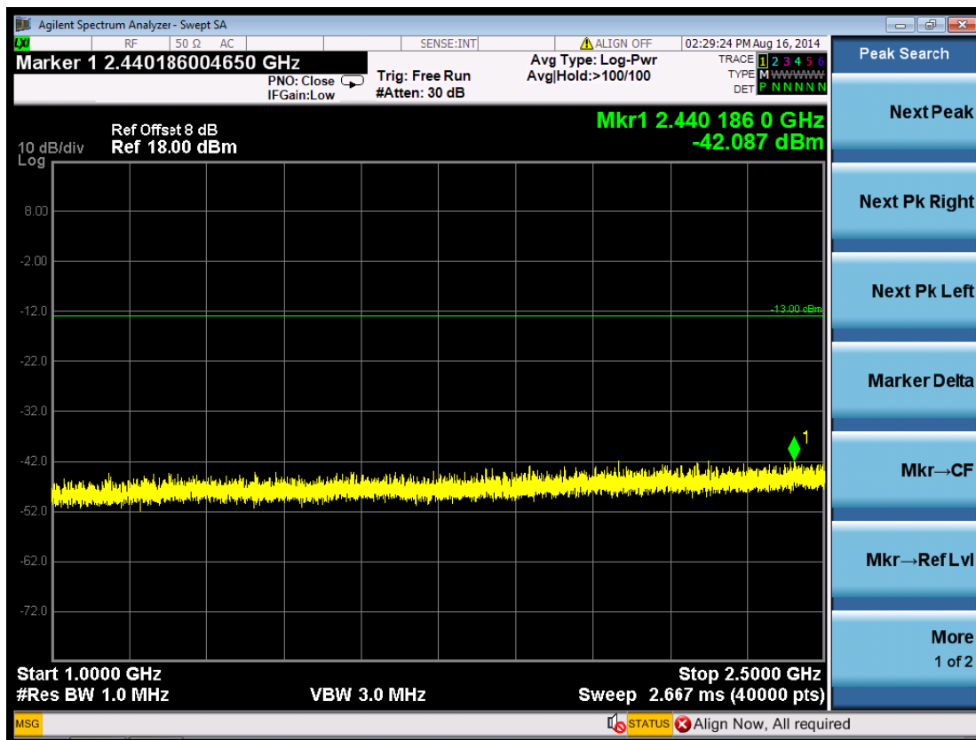
(Plot 5.5.1 D4: Idle WCDMA Band II)
