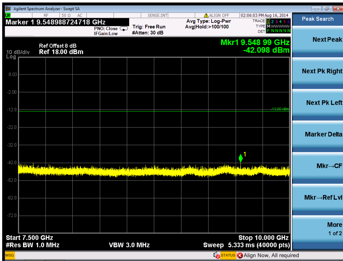
(Plot 5.5.3 D6: Idle WCDMA Band IV)
