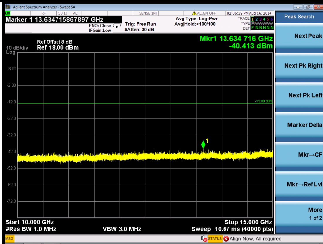
(Plot 5.5.3 D7: Idle WCDMA Band IV)
