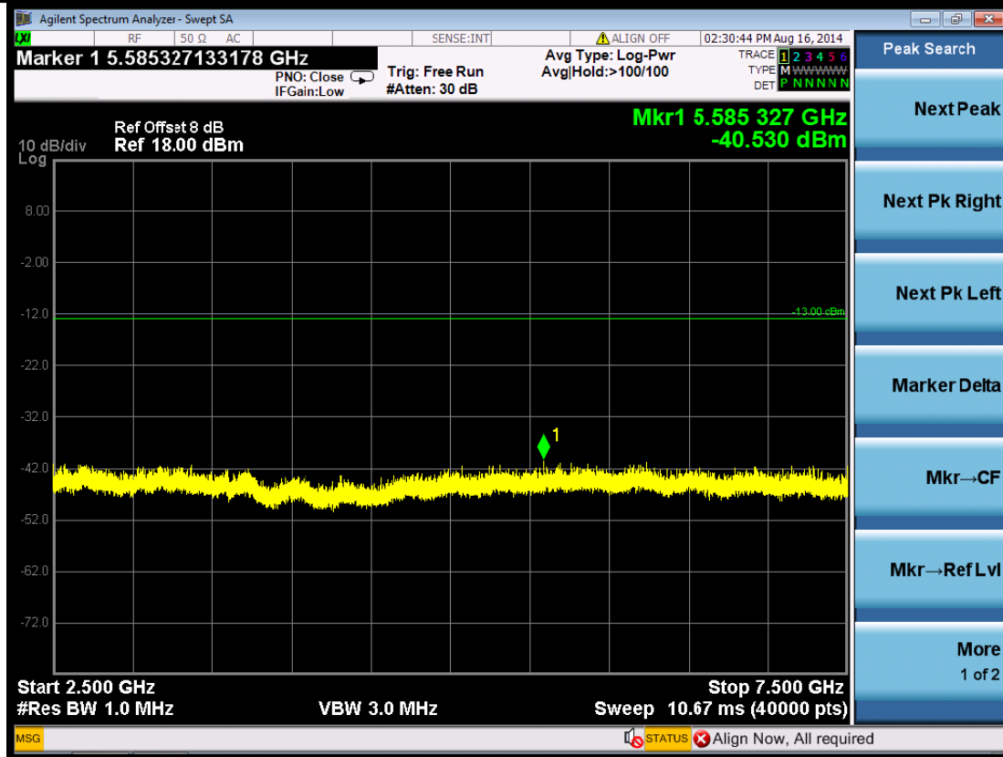
(Plot 5.5.1 D5: Idle WCDMA Band II)
