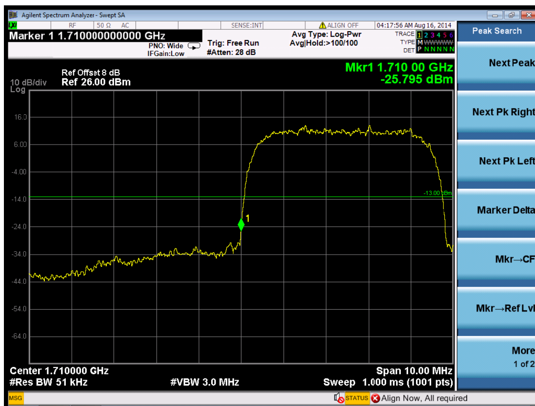
(Plot 5.4.2 A: Channel 1312: 1712.4MHz WCDMA Band IV)
