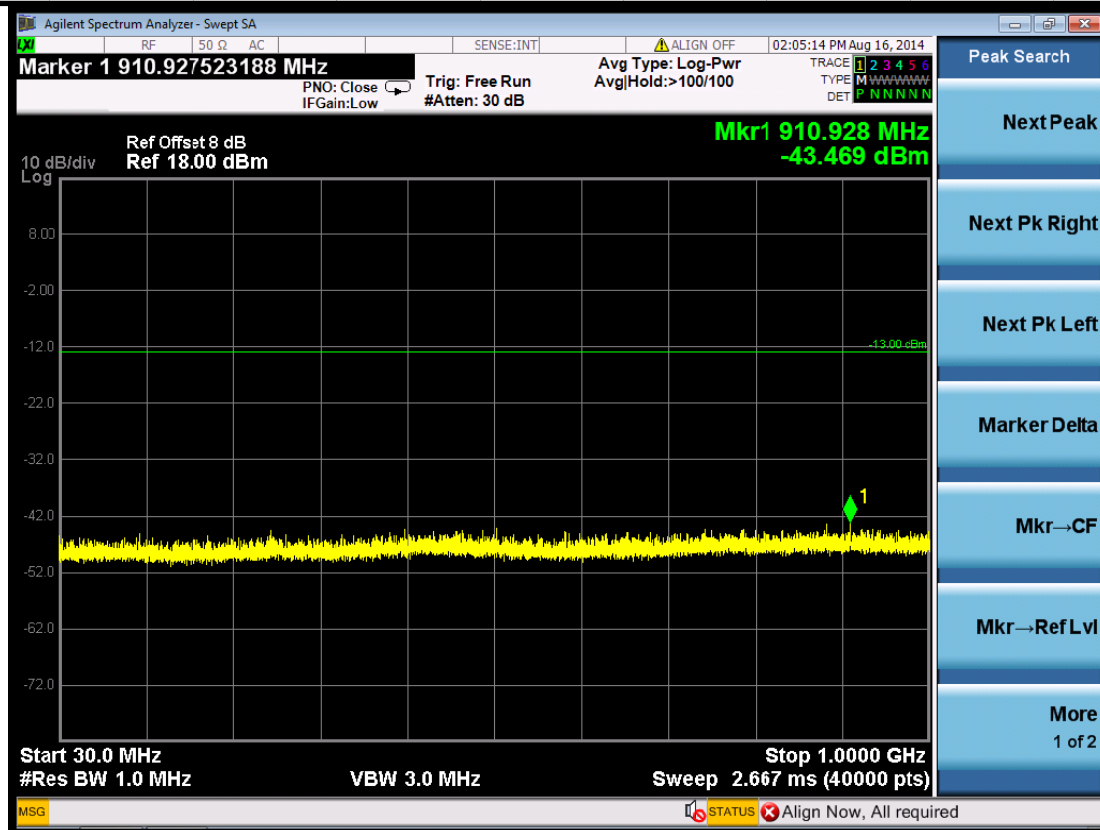
(Plot 5.5.3 D3: Idle WCDMA Band IV)
