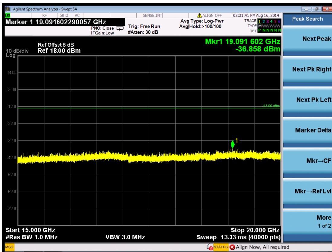
(Plot 5.5.1 D8: Idle WCDMA Band II)
