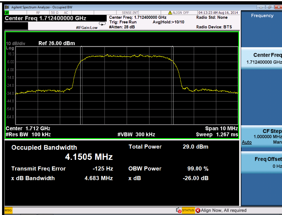
(Plot 5.3.2 A: Channel 1312: 1712.4MHz WCDMA Band IV)
