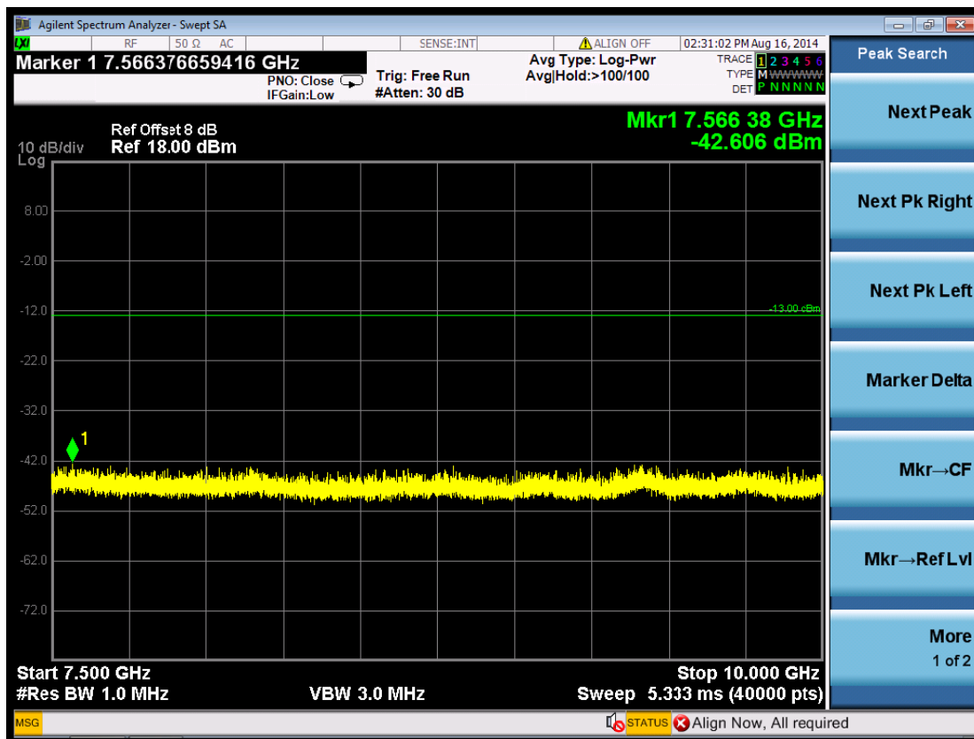
(Plot 5.5.1 D6: Idle WCDMA Band II)
