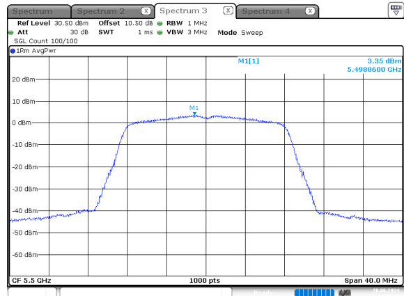
a_5500MHz_Chain 1
