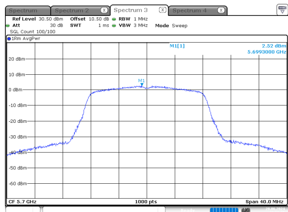
a_5700MHz_Chain 1
