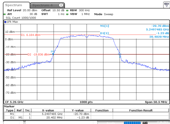
a_5260MHz_Chain 0
