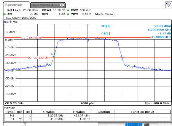
n40_5230MHz_Chain 0
