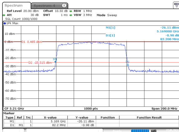
ac80_5210MHz_Chain 0
