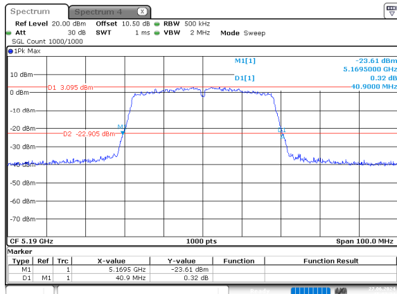
n40_5190MHz_Chain 0
