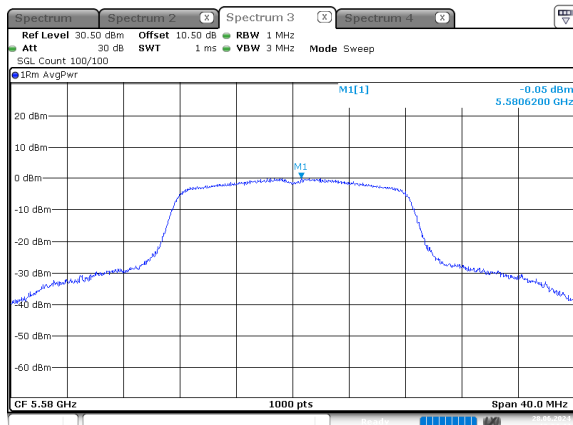
a_5580MHz_Chain 0
