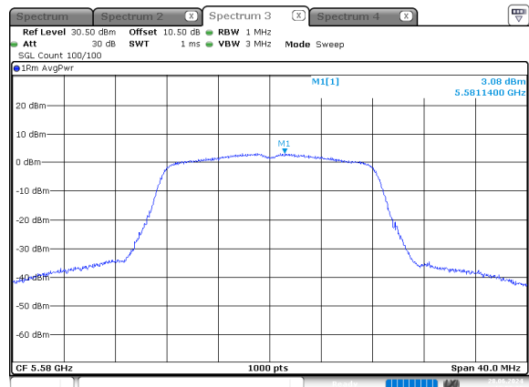
a_5580MHz_Chain 1
