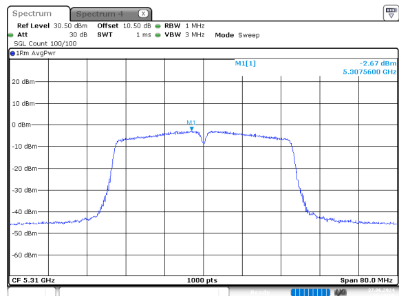
n40_5310MHz_Chain 1
