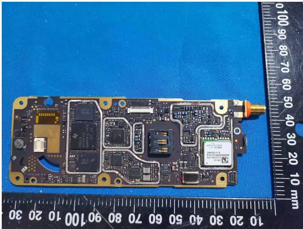
GPS Module
