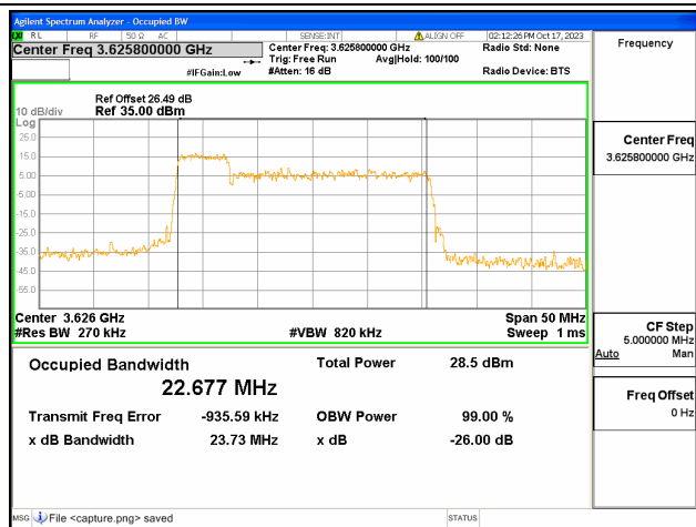
48C / 5+20MHz / QPSK/ Mid CH
