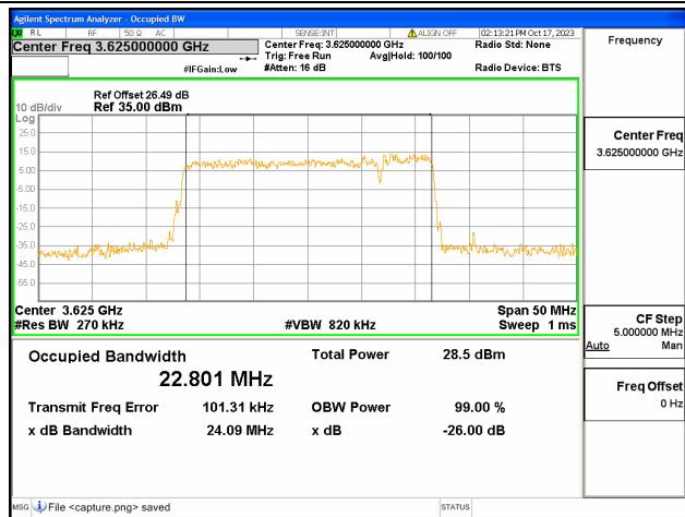
48C / 20+5MHz / QPSK/ Mid CH
