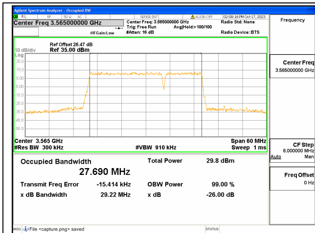
48C / 20+10MHz / QPSK/ Low CH
