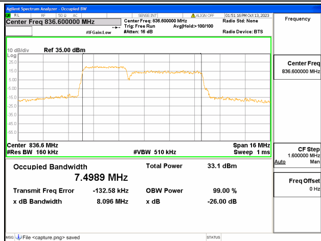
5B / 3+5MHz / QPSK/ Mid CH
