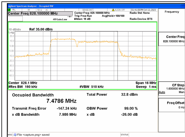
5B / 3+5MHz / QPSK/ Low CH
