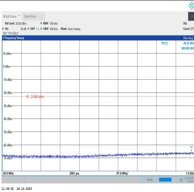
2-2-20MHz-20MHz-QPSK-QPSK-18801-18999-1RB#0-1RB#9 9-30~1000MHz-PASS
