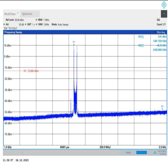
2-2-20MHz-20MHz-QPSK-QPSK-18801-18999-1RB#0-1RB#9 9-1000~3000MHz-PASS
