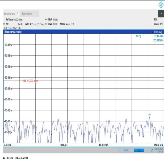
2-2-20MHz-20MHz-QPSK-QPSK-18801-18999-100RB#0-100 RB#0-0.009~0.15MHz-PASS
