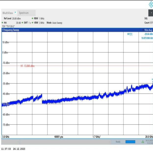
2-2-20MHz-20MHz-QPSK-QPSK-18801-18999-1RB#0-1RB#9 9-3000~20000MHz-PASS
