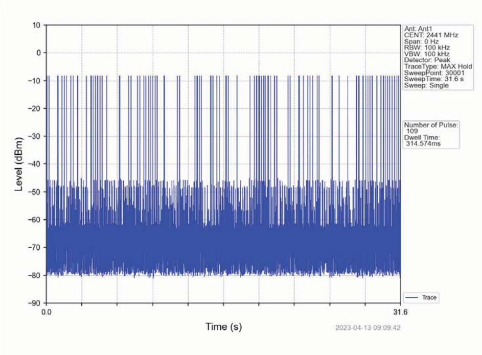
Pi/4DQPSK_2DH5_HOPP_Ant1_NTNV
