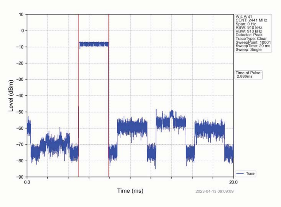
Pi/4DQPSK_2DH5_HOPP_Ant1_NTNV
