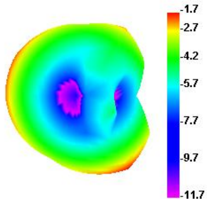
1710.000MHz
