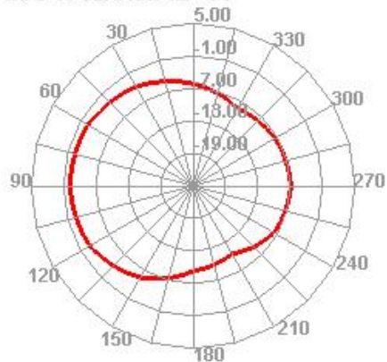
1851.428MHz H
