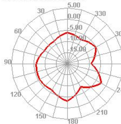
1851.428MHz E1
