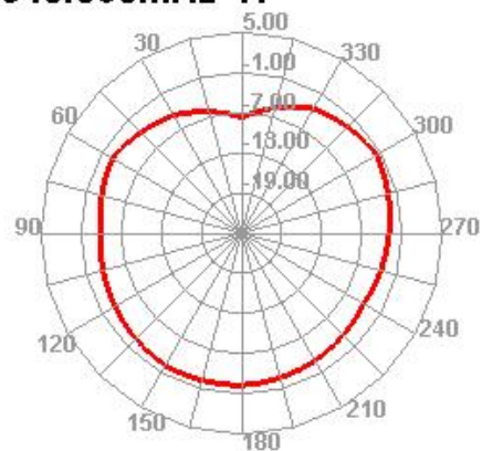
948.568MHz H
