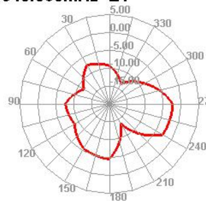
948.568MHz E1
