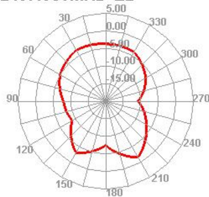
2497.956MHz E2
