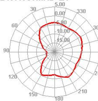
2497.956MHz E1
