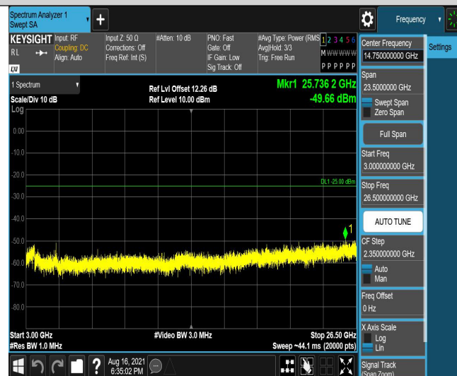
Band7-20MHz-QPSK-21350-100RB#0-Range3:3000~26500MHz
