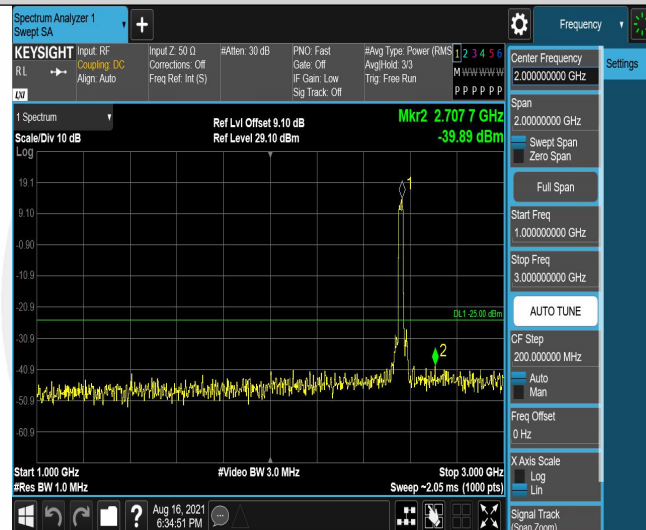
Band7-20MHz-QPSK-21350-100RB#0-Range2:1000~3000MHz
