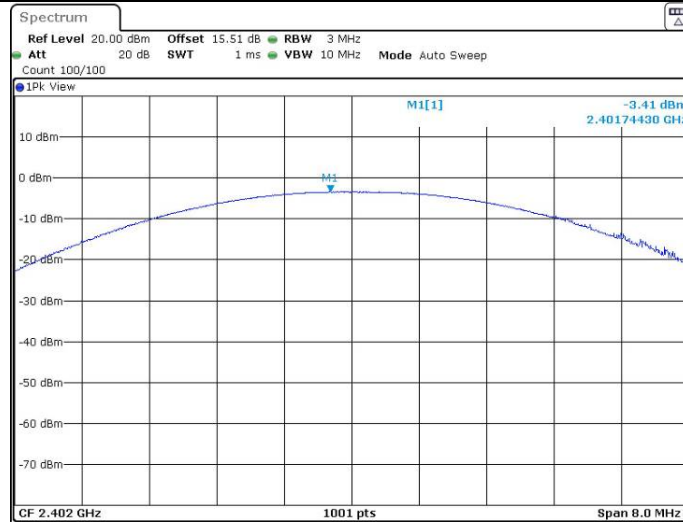
DH1_Ant1_2402
