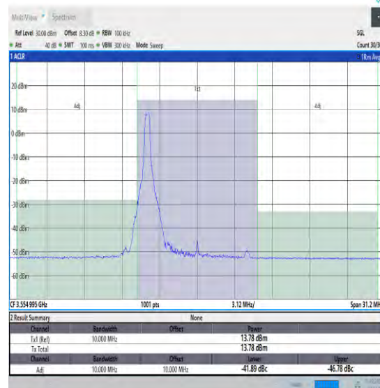
NTVN_N48_PC3_30_10_L_TID17_#1_-10_10
