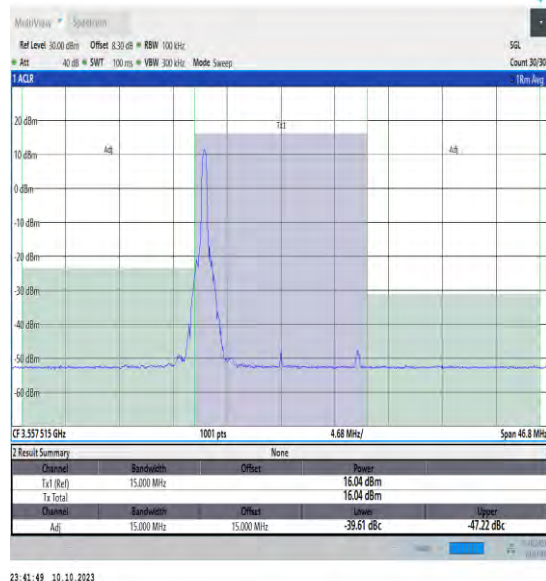
NTVN_N48_PC3_30_15_L_TID2_#1_-15_15
