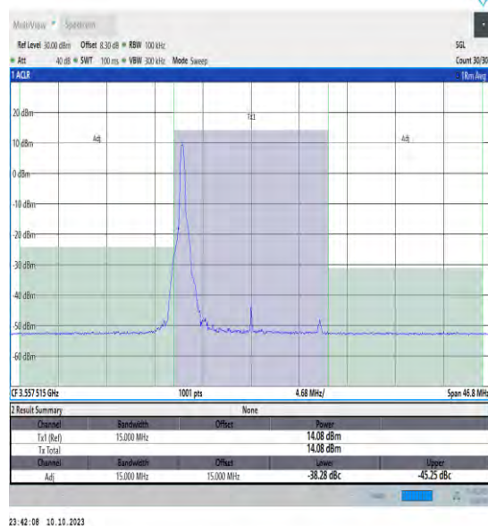
NTVN_N48_PC3_30_15_L_TID17_#1_-15_15
