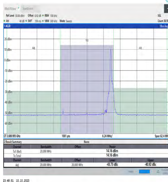
NTNV_N48_PC3_30_20_H_TID18_#1_-20_20
