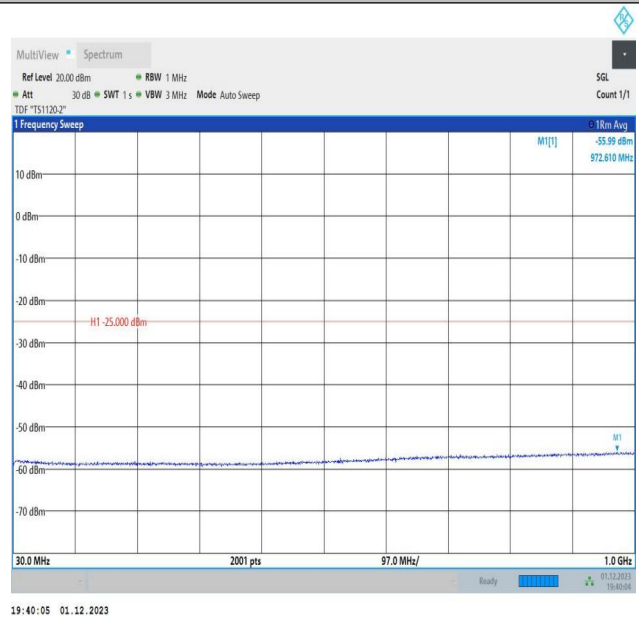
7-7-20MHz-15MHz-QPSK-QPSK-21026-21197-100RB#0-75R B#0-30~1000MHz-PASS
