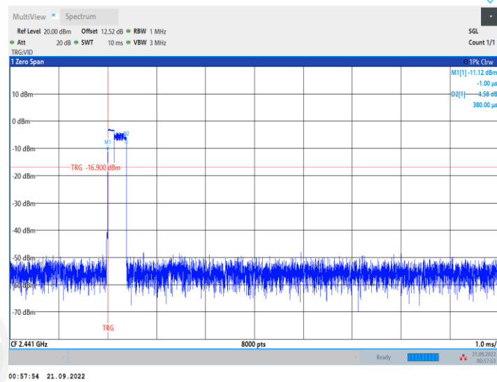
2DH1_Ant1_Hop
