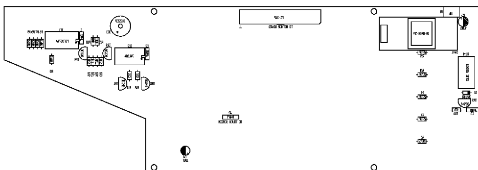
Bottom Layer
