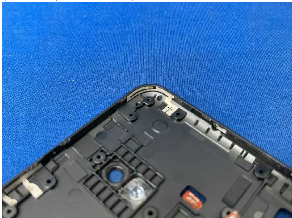
(26) EUT Photo (Antenna_WiFi & BT)
