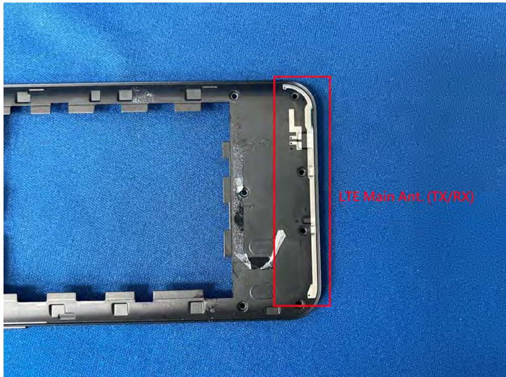
(29) EUT Photo (Antenna_LTE main)
