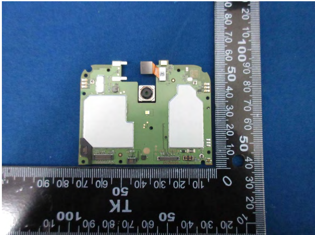
(10) EUT Photo
