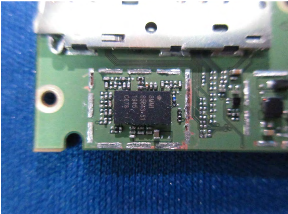
(16) EUT Photo
