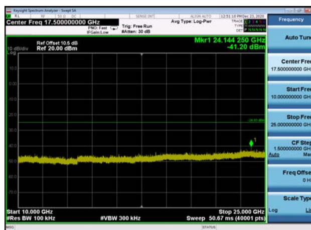
,Plot 5,10000MHz~25000MHz-802.11n(HT4 0) ,2452MHz
