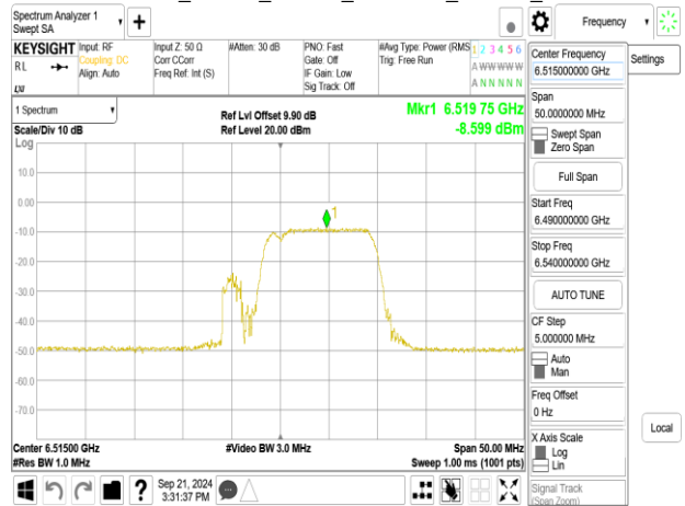
802.11be_20MHz_ChainA_6515MHz_52+26_MRU3
