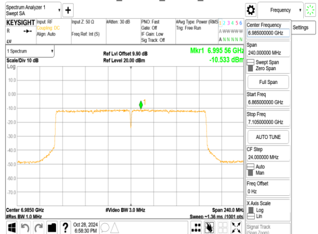
802.11ax_160MHz_ChainB_6985MHz_RU996_67
