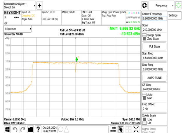
802.11ax_160MHz_ChainA_6665MHz_RU996_67
