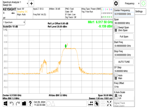
802.11be_20MHz_ChainA_6515MHz_RU106_54
