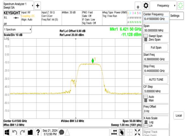
802.11be_20MHz_ChainA_6415MHz_RU26_8
