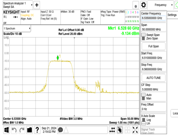
802.11be_20MHz_ChainA_6535MHz_RU106_53
