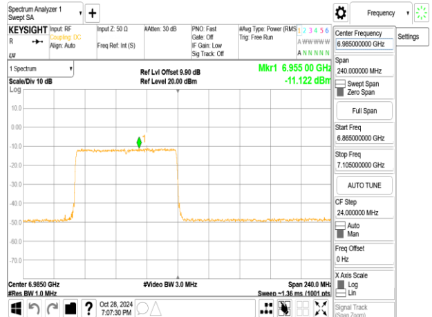
802.11ax_160MHz_ChainB_6985MHz_RU996_S67
