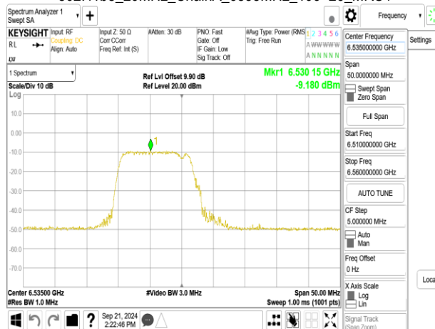
802.11be_20MHz_ChainA_6535MHz_52+26_MRUI
