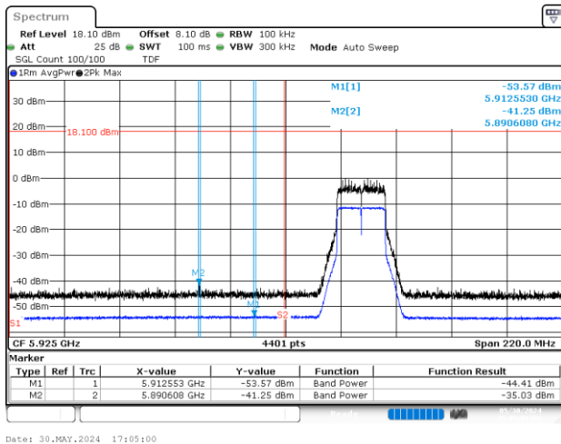
BE-NR-LOW, SISO-A, 802.11ax/be20-MCS0, Ch1
