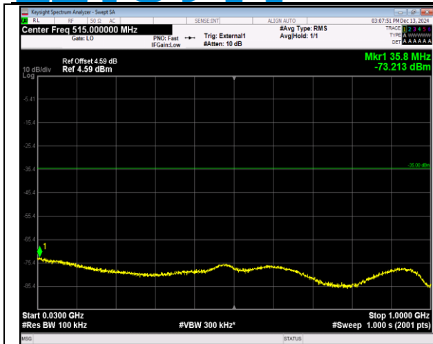
41(2555-2655)-41(2555-2655)-5MHz-20MHz-QPSK-QPS K-40273-40390-25RB#0-100RB#0-30~1000MHz-PASS
