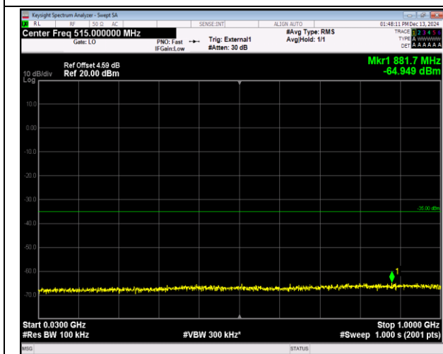
38-38-20MHz-20MHz-QPSK-QPSK-37901-38099-100RB#0-100RB#0-30~1000MHz-PASS
