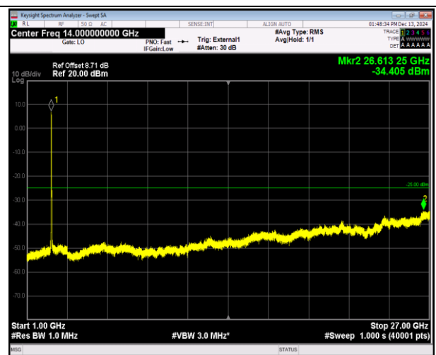
38-38-20MHz-20MHz-QPSK-QPSK-37901-38099-100RB#0-100RB#0-1000~27000MHz-PASS
