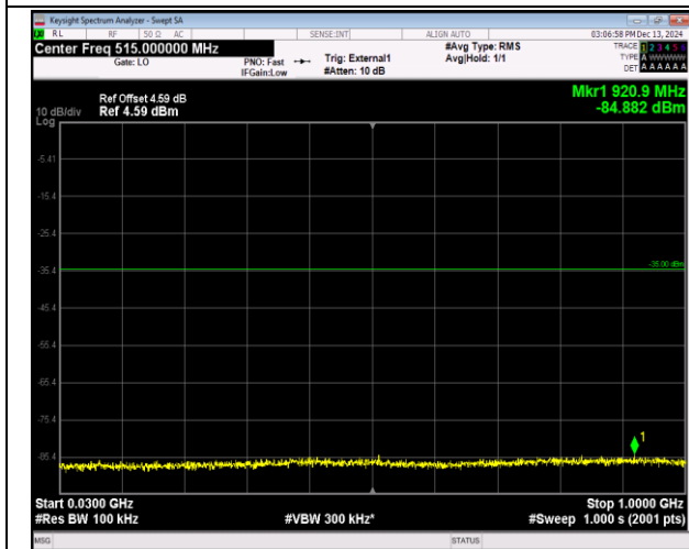
41(2555-2655)-41(2555-2655)-5MHz-20MHz-16QAM-16 QAM-40273-40390-1RB#0-1RB#99-30~1000MHz-PASS
