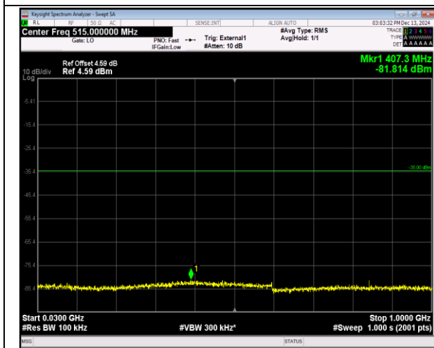
41(2555-2655)-41(2555-2655)-5MHz-20MHz-16QAM-16 QAM-40273-40390-1RB#0-0RB#0-30~1000MHz-PASS
