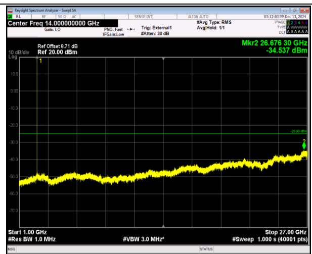
41(2555-2655)-41(2555-2655)-5MHz-20MHz-QPSK-QPSK- 40648-40765-1RB#24-0RB#0-1000~27000MHz-PASS
