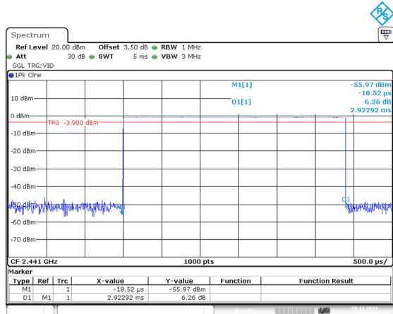
DH5_Hopping 2.923ms
