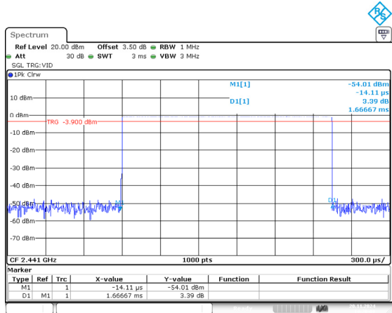
DH3_Hopping 1.667ms
