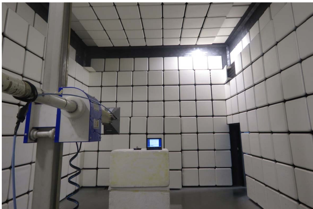
1GHz-18GHz
