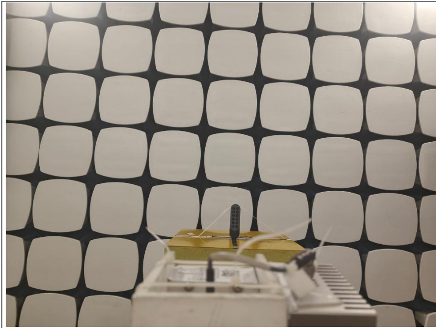
18GHz-26.5GHz
