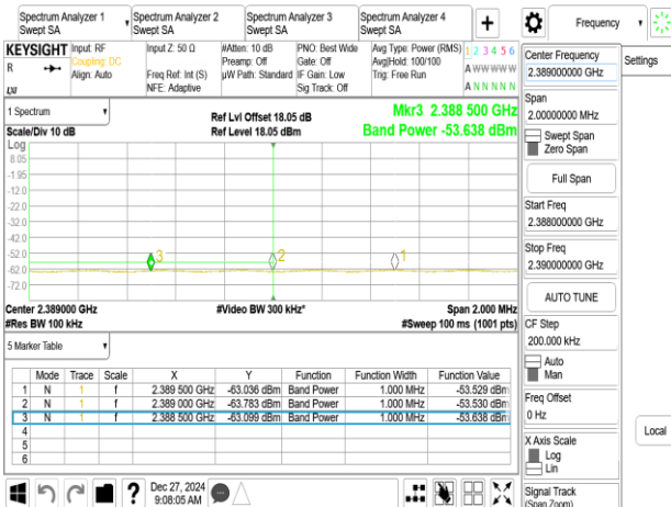
802.11g_20MHz_Chain0_2427MHz
