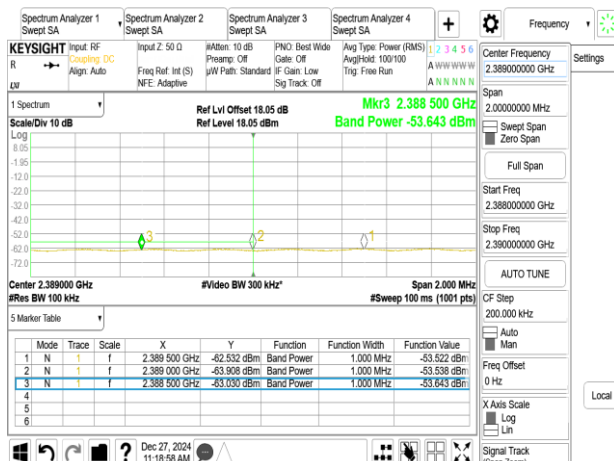
802.11n_20MHz_Chain1_2422MHz
