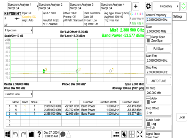
802.11g_20MHz_Chain1_2427MHz
