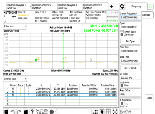
802.11g_20MHz_Chain0_2417MHz
