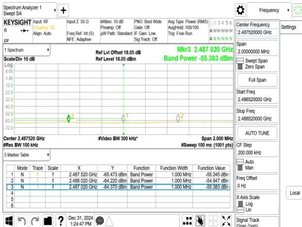
802.11b_20MHz_Chain1_2452MHz
