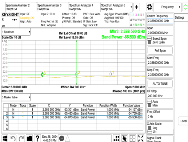
802.11g_20MHz_Chain1_2417MHz
