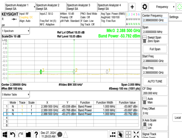
802.11n_20MHz_Chain0_2432MHz
