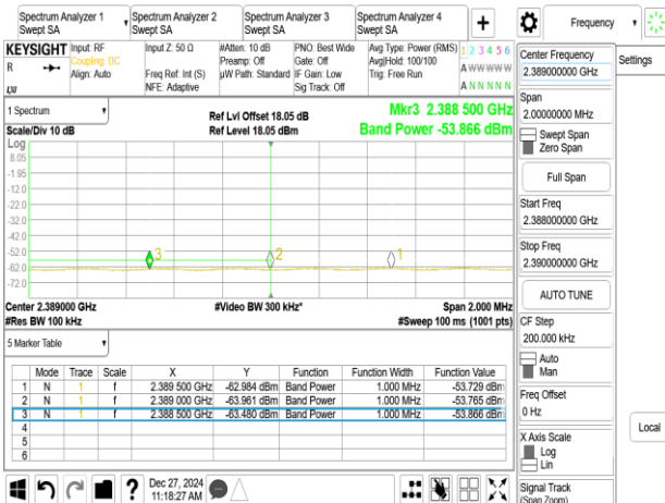
802.11n_20MHz_Chain0_2427MHz
