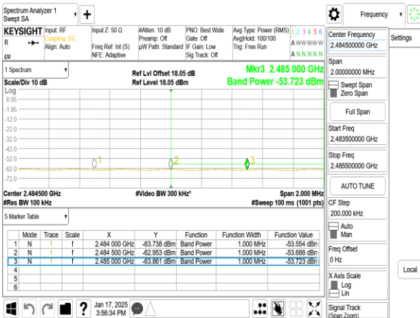
802.11g_20MHz_Chain1_2457MHz
