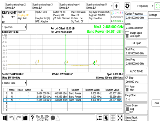
802.11b_20MHz_Chain1_2457MHz
