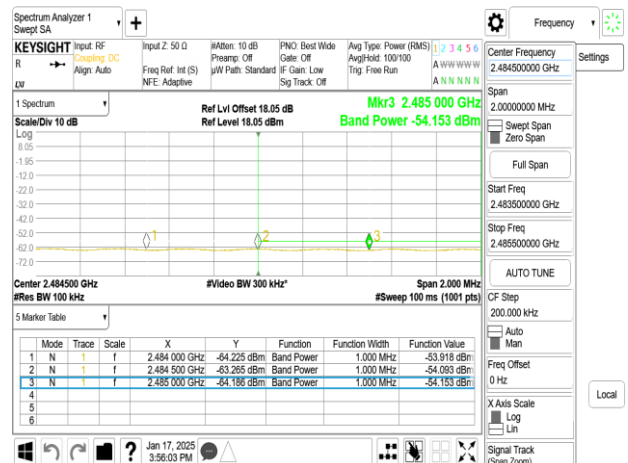
802.11g_20MHz_Chain0_2457MHz
