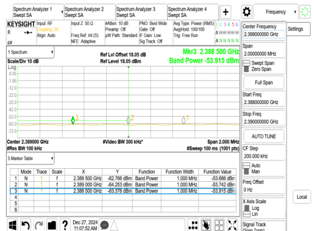
802.11n_20MHz_Chain0_2417MHz
