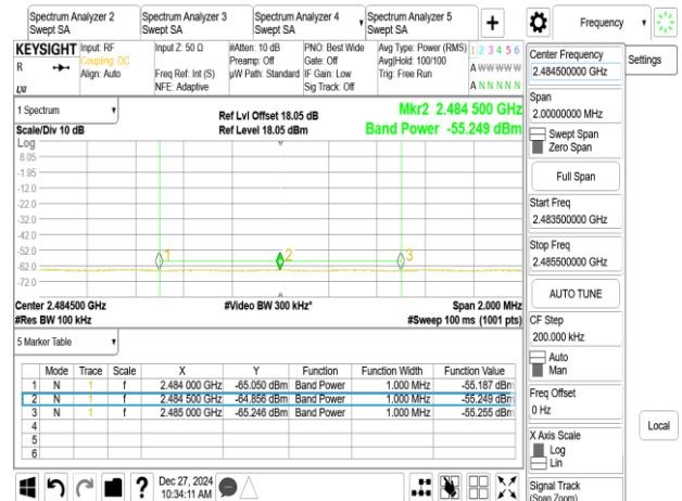
802.11g_20MHz_Chain0_2452MHz
