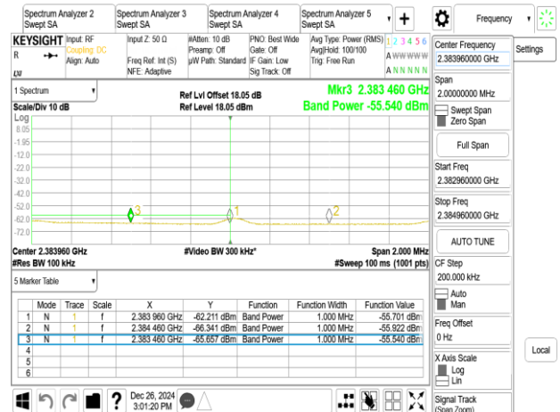
802.11b_20MHz_Chain1_2422MHz
