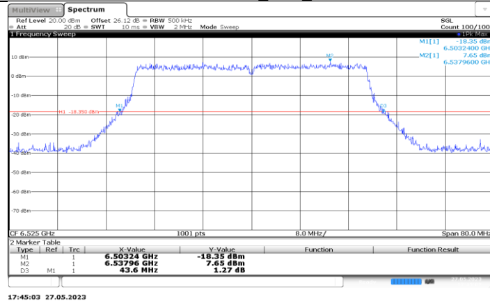
11AX40MIMO_Ant3_6525
