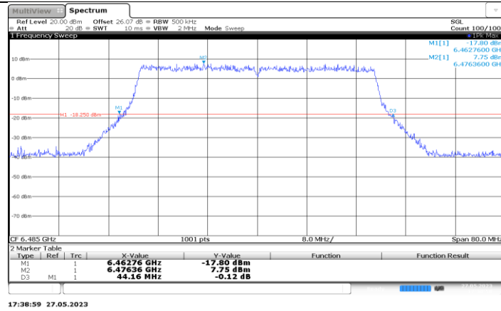
11AX40MIMO_Ant3_6485
