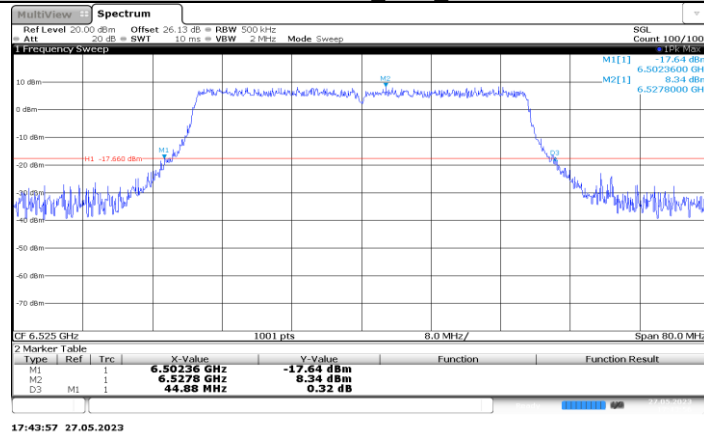
11AX40MIMO_Ant1_6525
