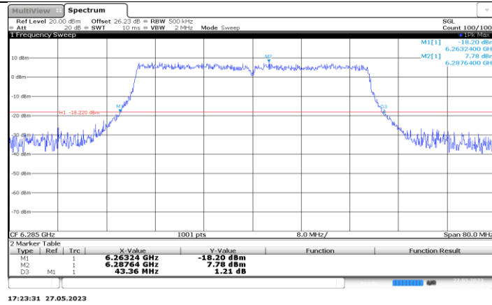
11AX40MIMO_Ant3_6285
