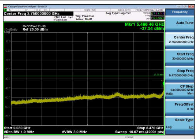
U-NII-2c ,Plot 2,30MHz~5470MHz-802.11 ax(40MHz),5510MHz,Ant0
