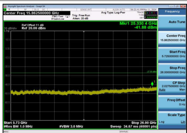
U-NII-2c ,Plot 3,5725MHz~26000MHz-802 .11ax(80MHz),5530MHz,Ant0
