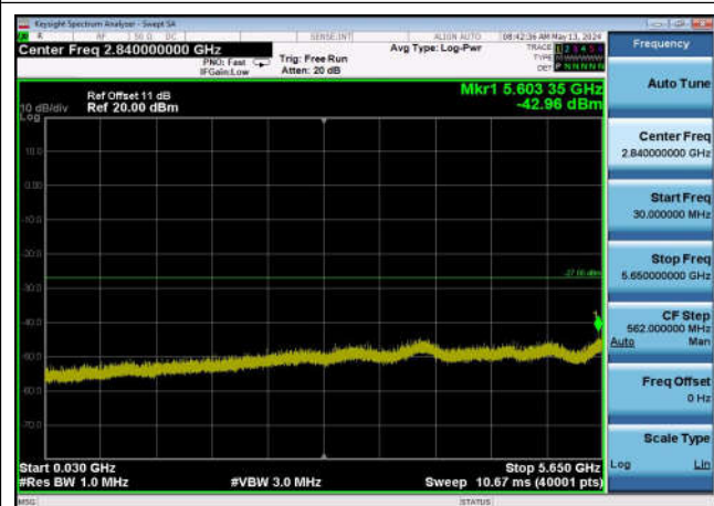
U-NII-3 ,Plot 2,30MHz~5650MHz-802.11a c(20MHz),5785MHz,Ant0
