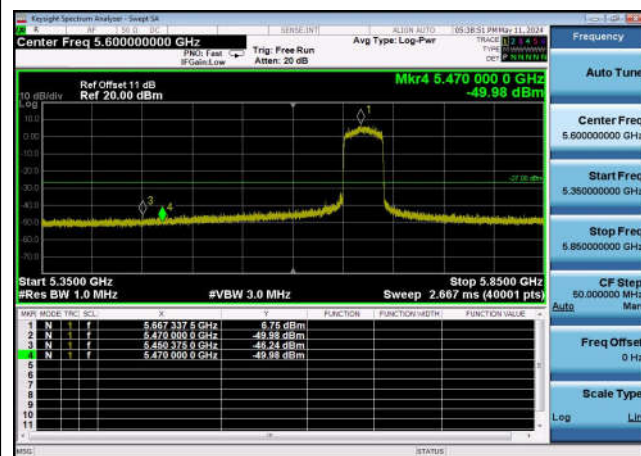
U-NII-2c ,Plot 1,Band Edge-802.11ax(8 0MHz),5610MHz,Ant0
