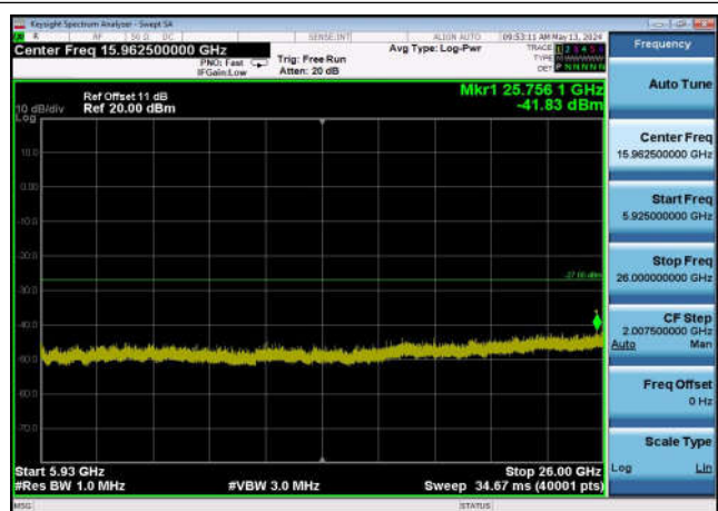
U-NII-3 ,Plot 3,5925MHz~26000MHz-802. 11ac(80MHz),5775MHz,Ant0
