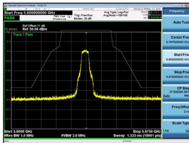
U-NII-3 ,Plot 1,Band Edge-802.11ac(40 MHz),5755MHz,Ant0
