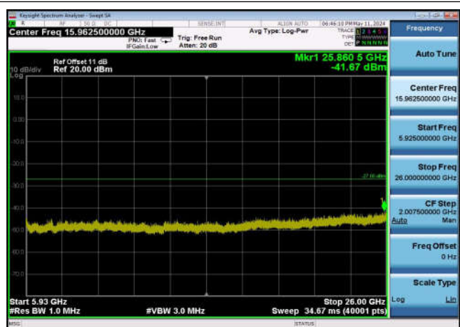
U-NII-3 ,Plot 3,5925MHz~26000MHz-802.11a(20MHz),5825MHz,Ant0
