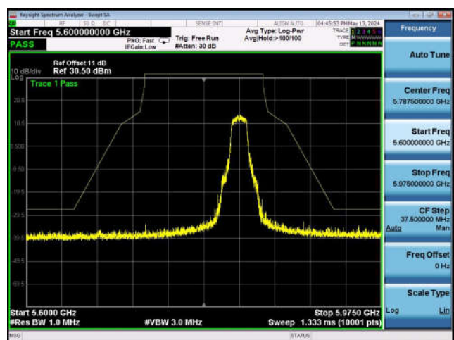
U-NII-3 ,Plot 1,Band Edge-802.11a(20MHz),5825MHz,Ant0
