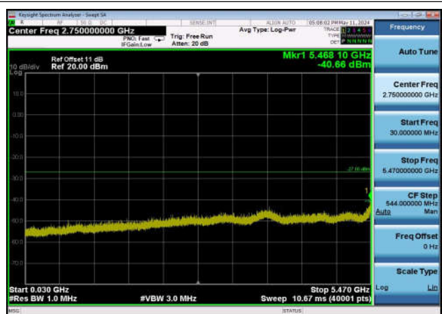
U-NII-2c ,Plot 2,30MHz~5470MHz-802.11 ac(40MHz),5670MHz,Ant0
