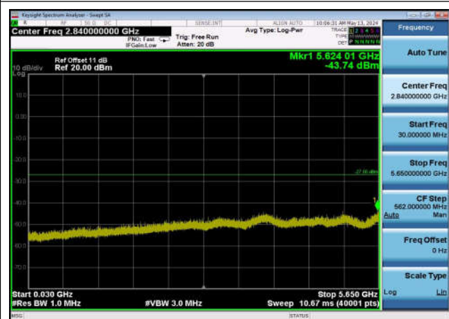
U-NII-3 ,Plot 2,30MHz~5650MHz-802.11a x(80MHz),5775MHz,Ant0
