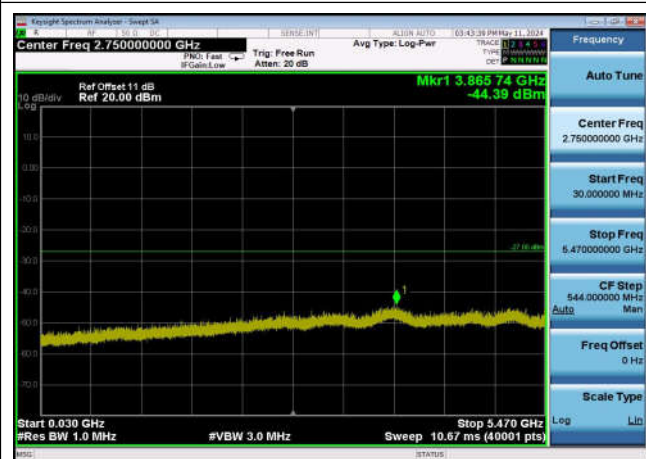
U-NII-2c ,Plot 2,30MHz~5470MHz-802.11 ac(40MHz),5590MHz,Ant0
