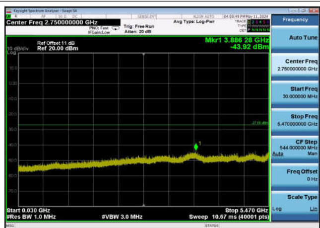
U-NII-2c ,Plot 2,30MHz~5470MHz-802.11 ax(40MHz),5510MHz,Ant0
