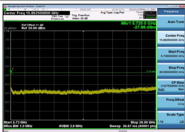
U-NII-2c ,Plot 3,5725MHz~26000MHz-802 .11ac(20MHz),5600MHz,Ant0
