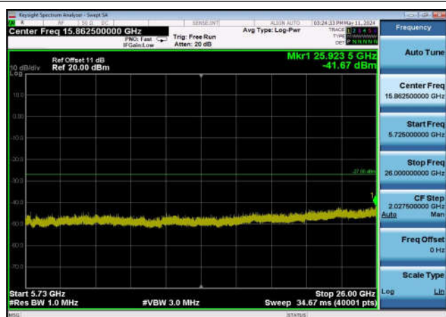
U-NII-2c ,Plot 3,5725MHz~26000MHz-802 .11ac(20MHz),5700MHz,Ant0
