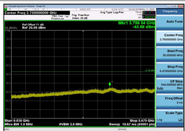
U-NII-2c ,Plot 2,30MHz~5470MHz-802.11 a(20MHz),5700MHz,Ant0
