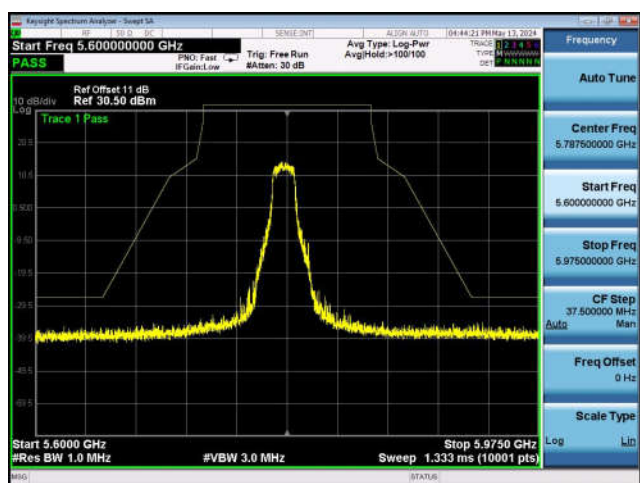
U-NII-3 ,Plot 1,Band Edge-802.11a(20MHz),5785MHz,Ant0
