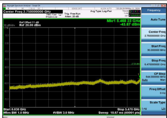
U-NII-2c ,Plot 2,30MHz~5470MHz-802.11 ac(40MHz),5510MHz,Ant0
