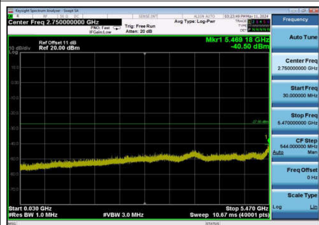
U-NII-2c ,Plot 2,30MHz~5470MHz-802.11 ac(20MHz),5700MHz,Ant0
