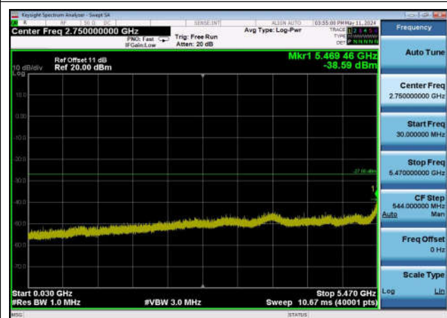
U-NII-2c ,Plot 2,30MHz~5470MHz-802.11 ax(20MHz),5700MHz,Ant0
