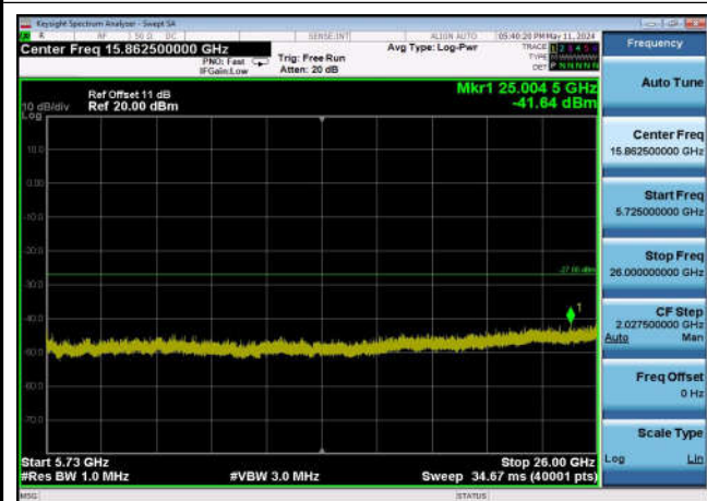
U-NII-2c ,Plot 3,5725MHz~26000MHz-802 .11ax(80MHz),5610MHz,Ant0
