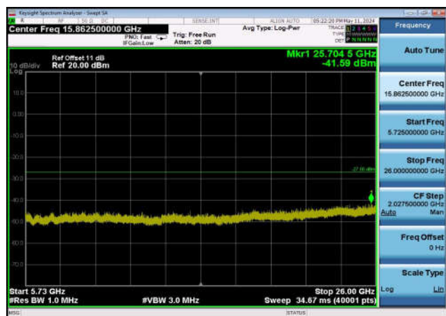
U-NII-2c ,Plot 3,5725MHz~26000MHz-802 .11ac(80MHz),5610MHz,Ant0
