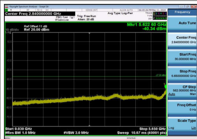
U-NII-3 ,Plot 2,30MHz~5650MHz-802.11a (20MHz),5825MHz,Ant0
