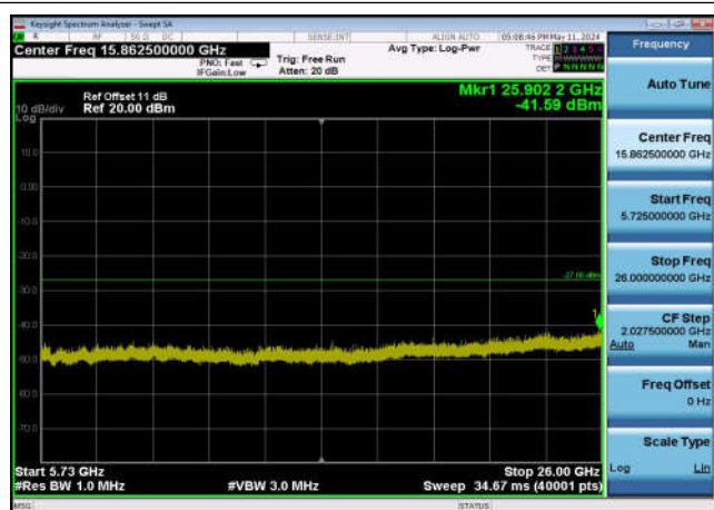
U-NII-2c ,Plot 3,5725MHz~26000MHz-802 .11ac(40MHz),5510MHz,Ant0
