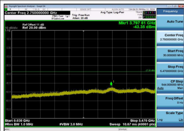
U-NII-2c ,Plot 2,30MHz~5470MHz-802.11 ax(20MHz),5700MHz,Ant0
