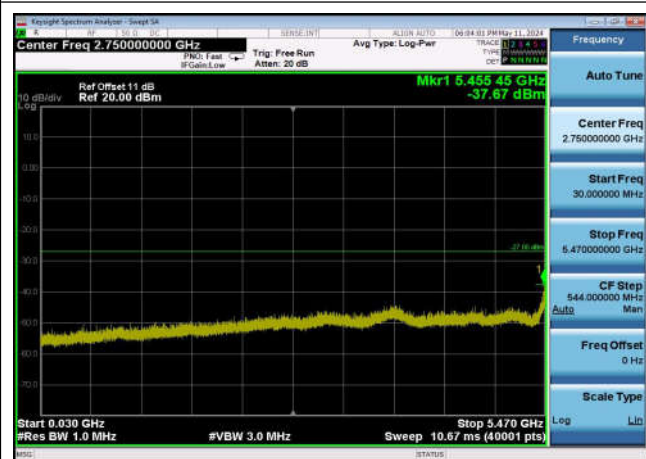
U-NII-2c ,Plot 2,30MHz~5470MHz-802.11 ax(20MHz),5500MHz,Ant0
