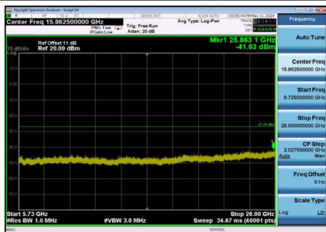
U-NII-2c ,Plot 3,5725MHz~26000MHz-802 .11ax(20MHz),5700MHz,Ant0
