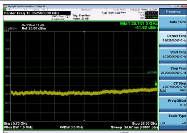
U-NII-2c ,Plot 3,5725MHz~26000MHz-802 .11ac(40MHz),5510MHz,Ant0
