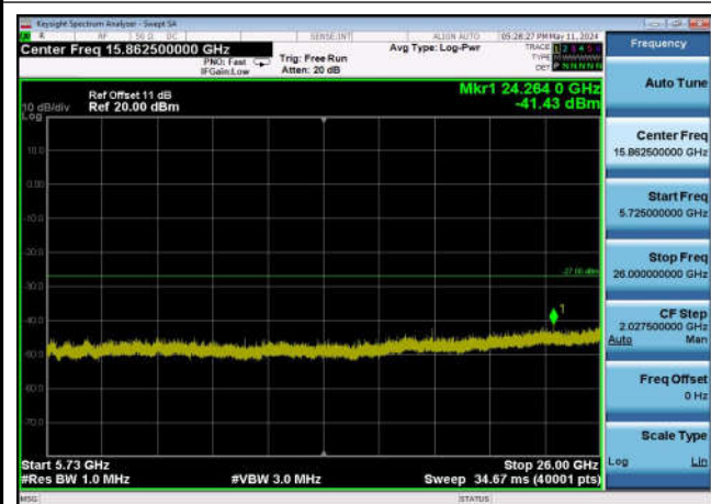
U-NII-2c ,Plot 3,5725MHz~26000MHz-802 .11ax(40MHz),5670MHz,Ant0
