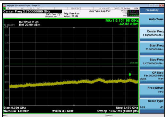
U-NII-2c ,Plot 2,30MHz~5470MHz-802.11 ac(40MHz),5670MHz,Ant0
