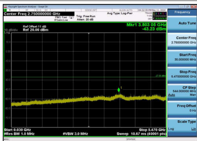
U-NII-2c ,Plot 2,30MHz~5470MHz-802.11 n(40MHz),5670MHz,Ant0
