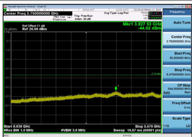
U-NII-2c ,Plot 2,30MHz~5470MHz-802.11 ax(80MHz),5610MHz,Ant0
