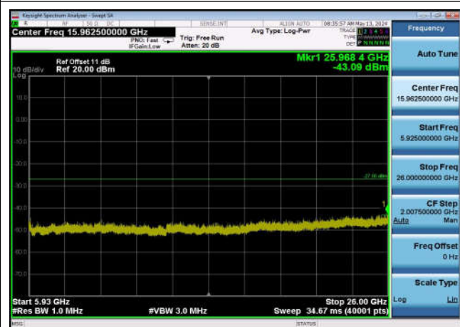
U-NII-3 ,Plot 3,5925MHz~26000MHz-802. 11ac(20MHz),5825MHz,Ant0
