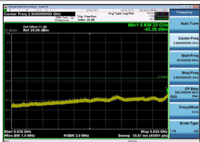
U-NII-3 ,Plot 2,30MHz~5650MHz-802.11a c(20MHz),5745MHz,Ant0
