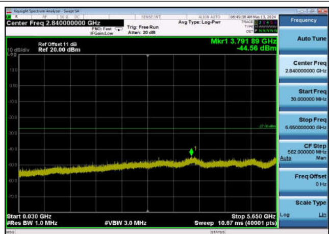
U-NII-3 ,Plot 2,30MHz~5650MHz-802.11a c(20MHz),5825MHz,Ant0
