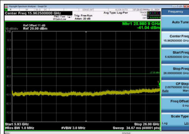
U-NII-3 ,Plot 3,5925MHz~26000MHz-802. 11n(20MHz),5825MHz,Ant0
