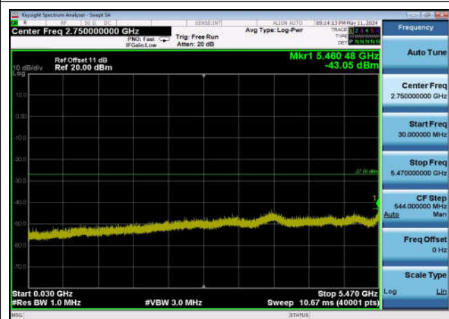
U-NII-2c ,Plot 2,30MHz~5470MHz-802.11 ac(40MHz),5590MHz,Ant0
