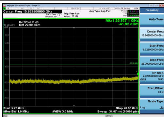
U-NII-2c ,Plot 3,5725MHz~26000MHz-802 .11ac(40MHz),5590MHz,Ant0
