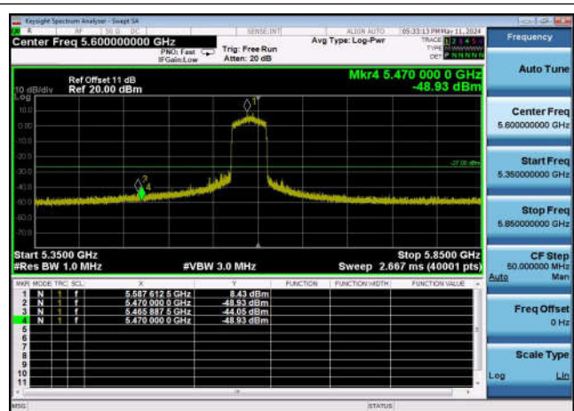
U-NII-2c ,Plot 1,Band Edge-802.11ax(4 0MHz),5590MHz,Ant0
