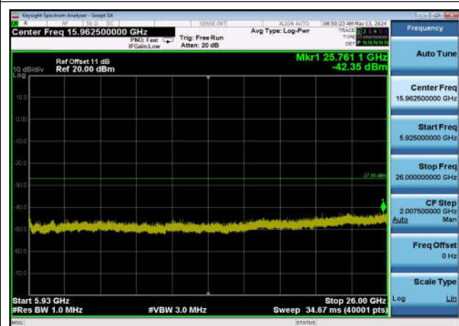
U-NII-3 ,Plot 3,5925MHz~26000MHz-802. 11ac(40MHz),5795MHz,Ant0
