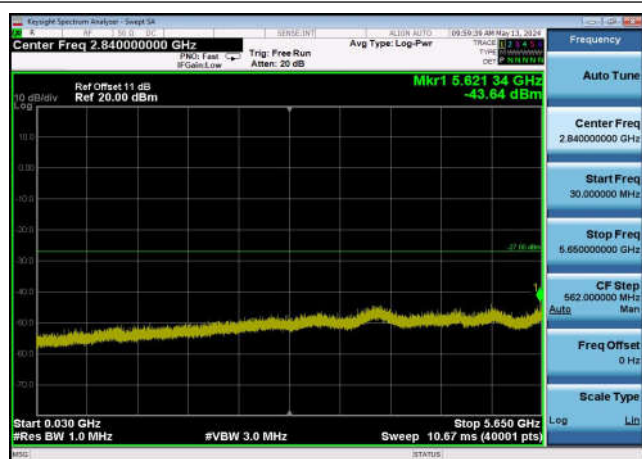
U-NII-3 ,Plot 2,30MHz~5650MHz-802.11a x(20MHz),5745MHz,Ant0
