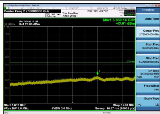
U-NII-2c ,Plot 2,30MHz~5470MHz-802.11 ax(80MHz),5530MHz,Ant0
