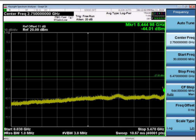
U-NII-2c ,Plot 2,30MHz~5470MHz-802.11 ax(20MHz),5600MHz,Ant0
