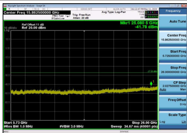
U-NII-2c ,Plot 3,5725MHz~26000MHz-802 .11ax(20MHz),5600MHz,Ant0
