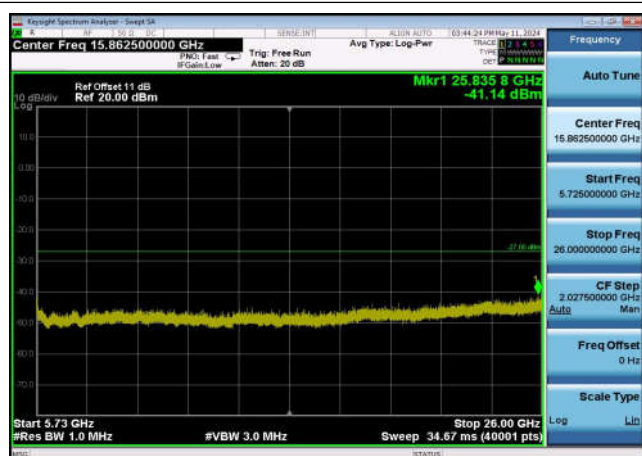
U-NII-2c ,Plot 3,5725MHz~26000MHz-802 .11ac(40MHz),5590MHz,Ant0
