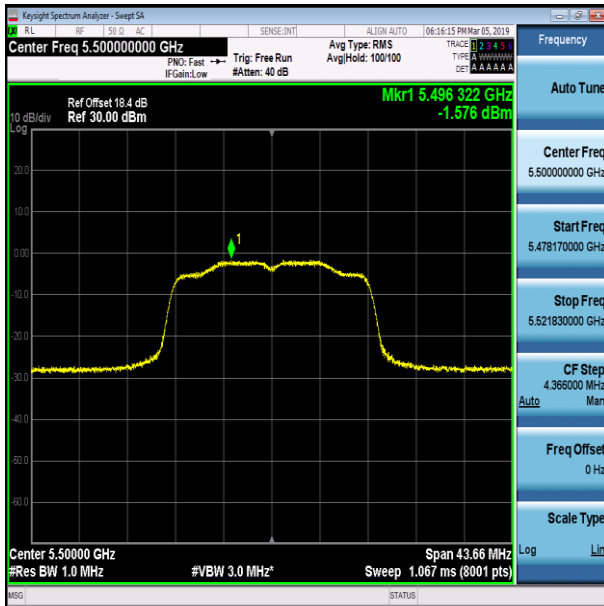
11A-Ant1-5500
