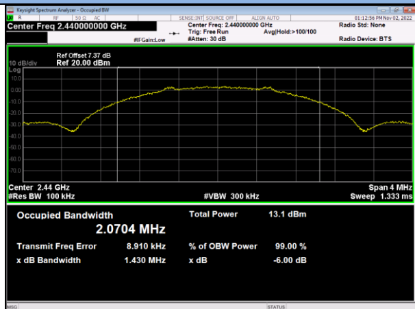
2Mbps / 2440MHz
