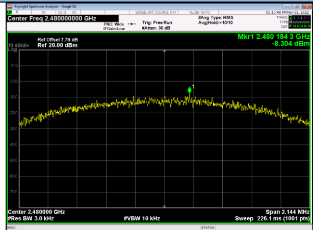
2Mbps / 2480MHz
