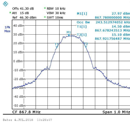
Figure 80. — 867.8MHz GSM Input
