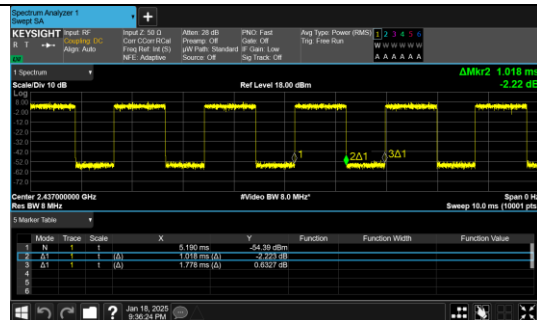
IEEE 802.11ax 20MHz Channel 6
