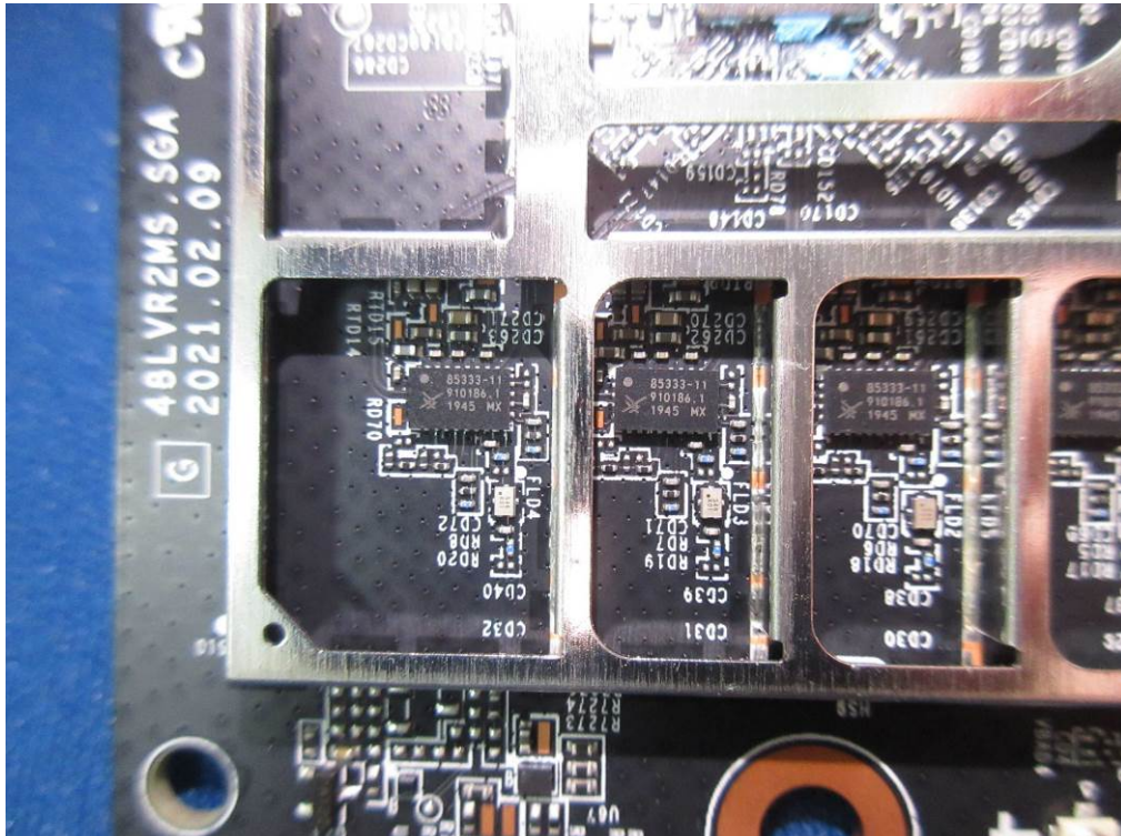
(87) EUT Photo
