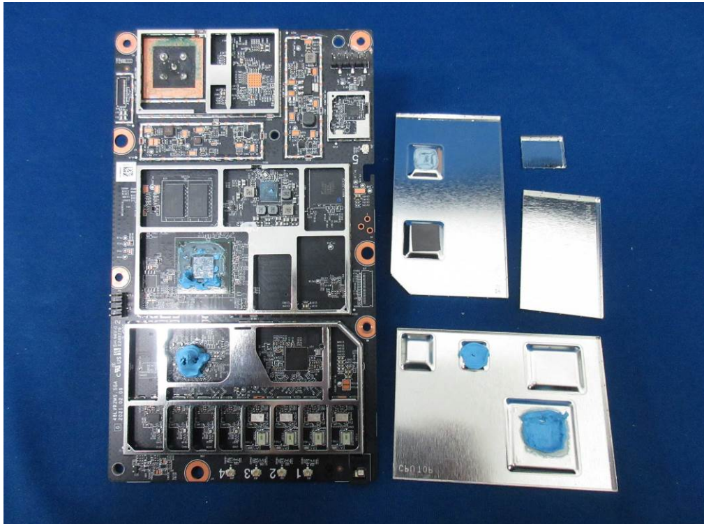
(71) EUT Photo
