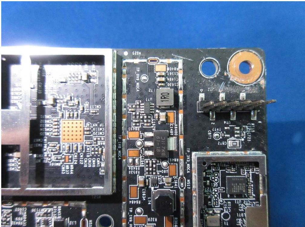
(75) EUT Photo
