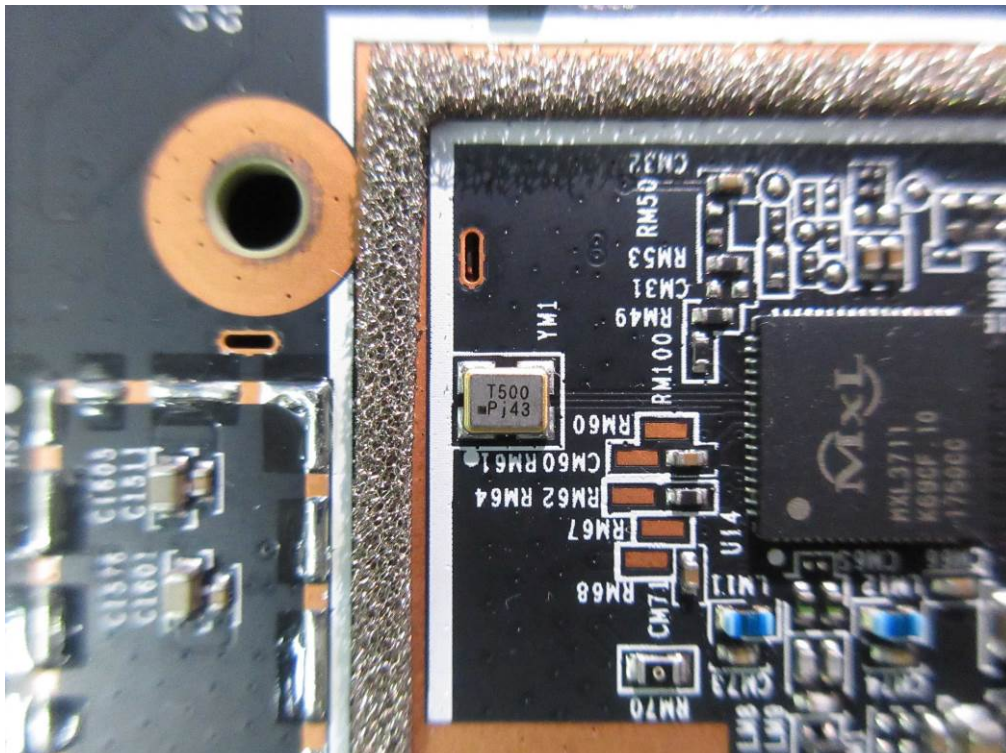
(69) EUT Photo
