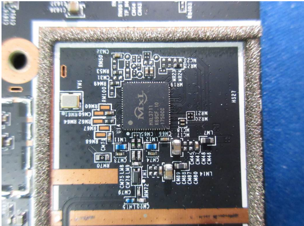
(67) EUT Photo
