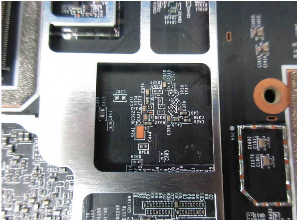
(65) EUT Photo
