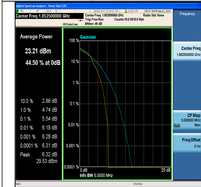
Band2-5MHz-16QAM-18625-1RB#0-PASS
