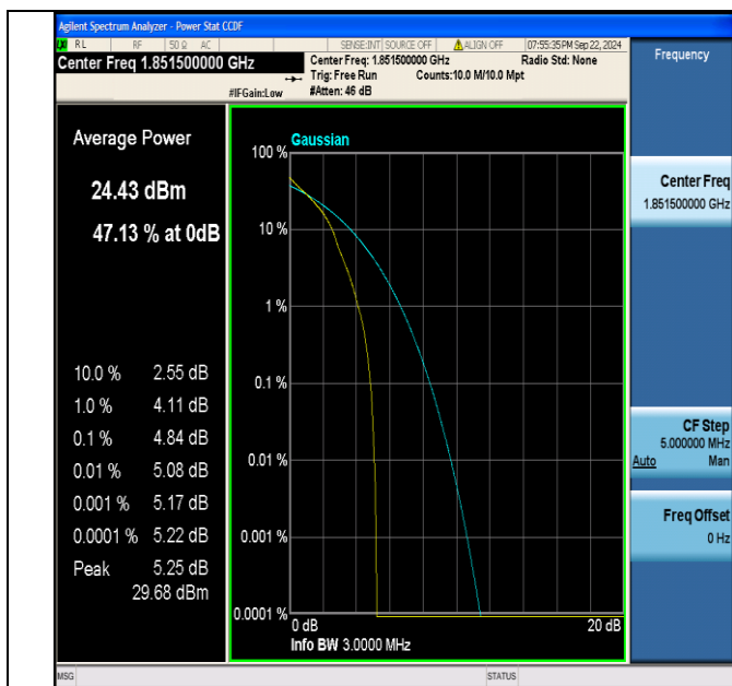
Band2-3MHz-QPSK-18615-1RB#0-PASS
