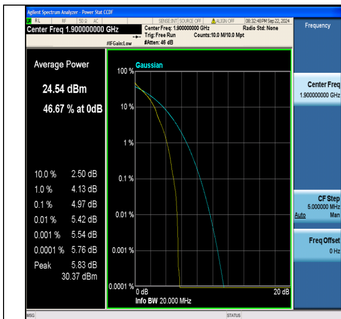
Band2-20MHz-QPSK-19100-1RB#0-PASS
