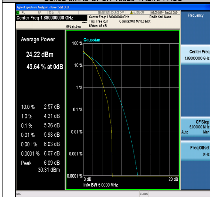
Band2-5MHz-QPSK-18900-1RB#0-PASS
