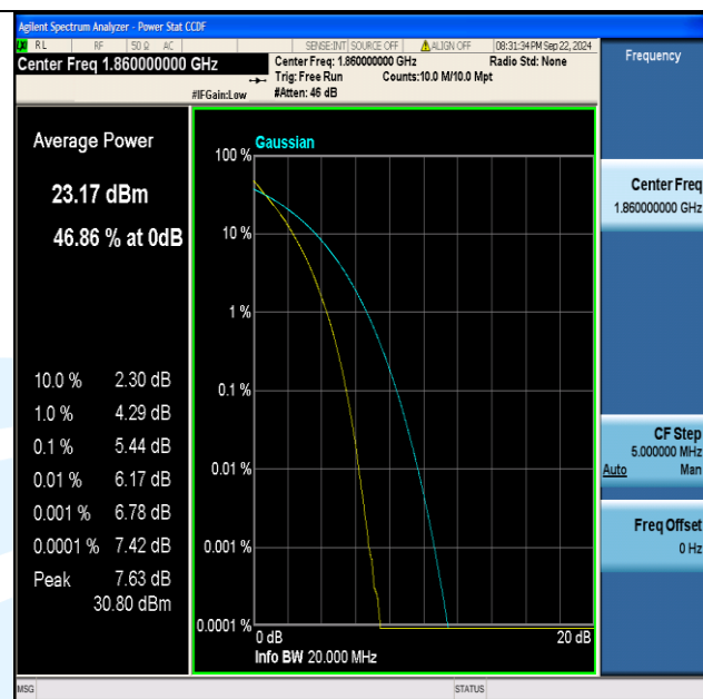
Band2-20MHz-QPSK-18700-100RB#0-PASS
