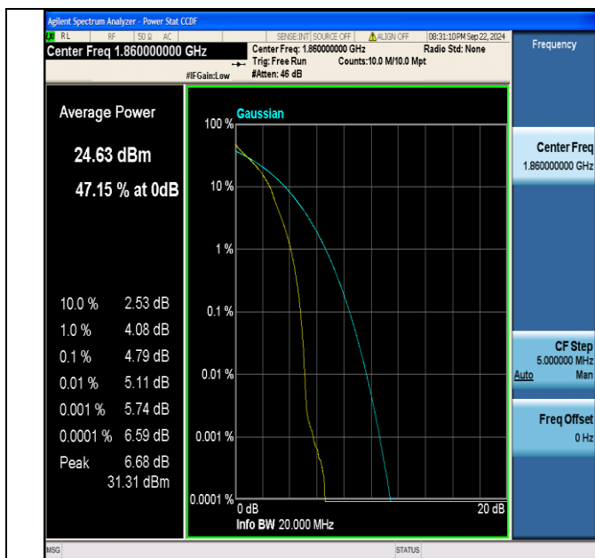
Band2-20MHz-QPSK-18700-1RB#0-PASS
