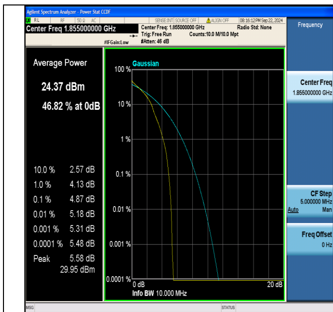
Band2-10MHz-QPSK-18650-1RB#0-PASS
