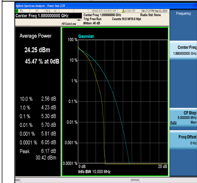
Band2-10MHz-QPSK-18900-1RB#0-PASS
