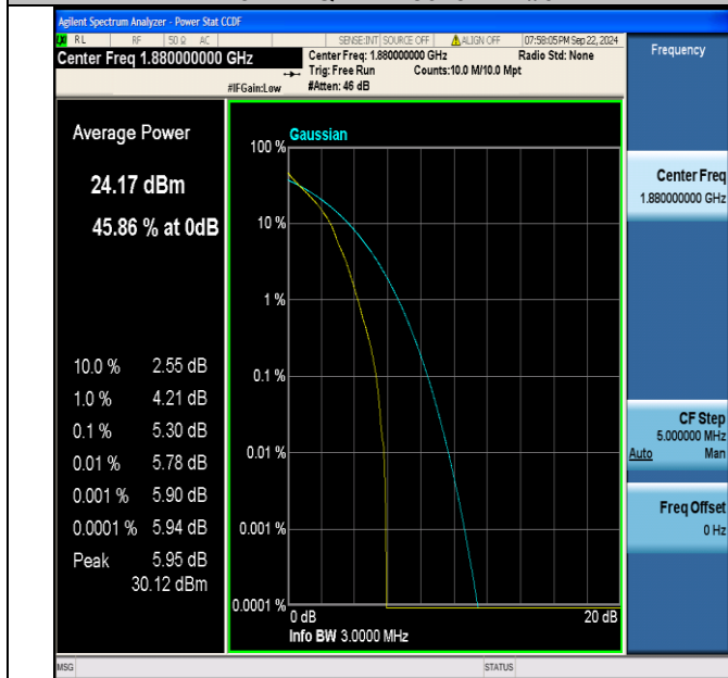
Band2-3MHz-QPSK-18900-1RB#0-PASS
