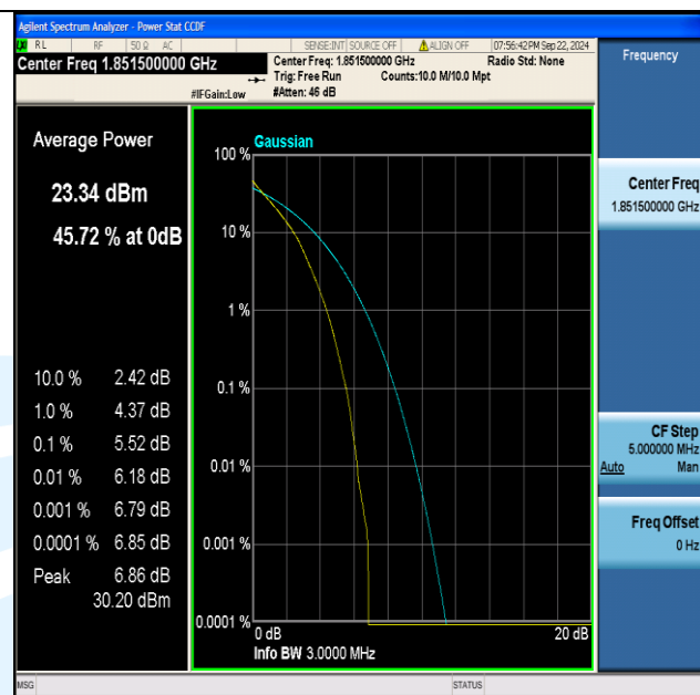
Band2-3MHz-QPSK-18615-15RB#0-PASS
