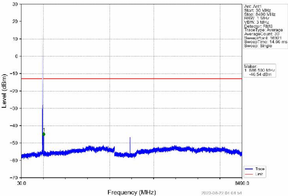
Band5_10MHz_QPSK_HCH_844MHz_RB_1_49_NTNV
