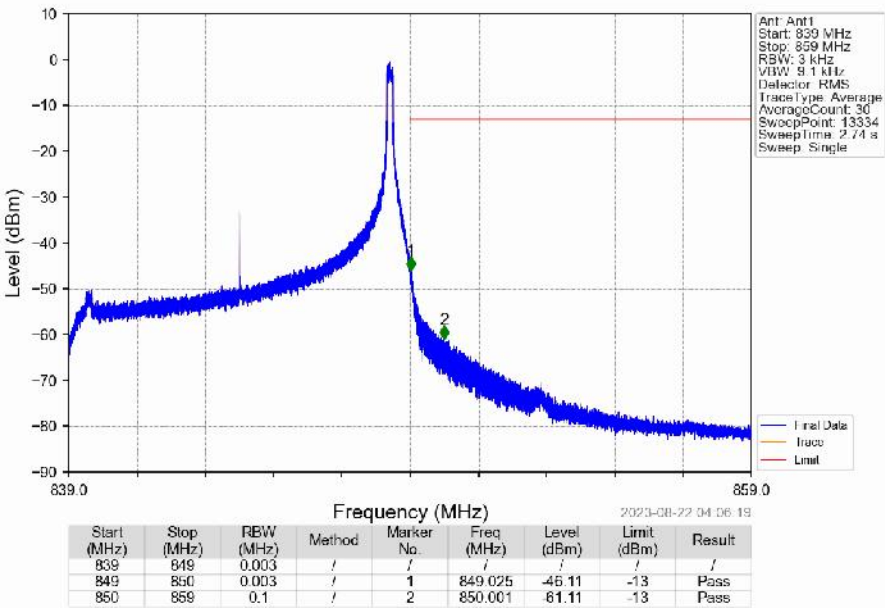
Band5_10MHz_QPSK_HCH_844MHz_RB_1_49_NTNV
