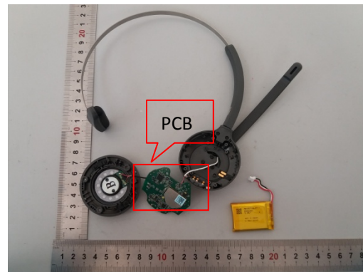
CP-HS-WL-561-N-US -PCB
